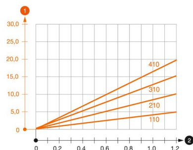
Belastingsdiagram console type MWAG 12
