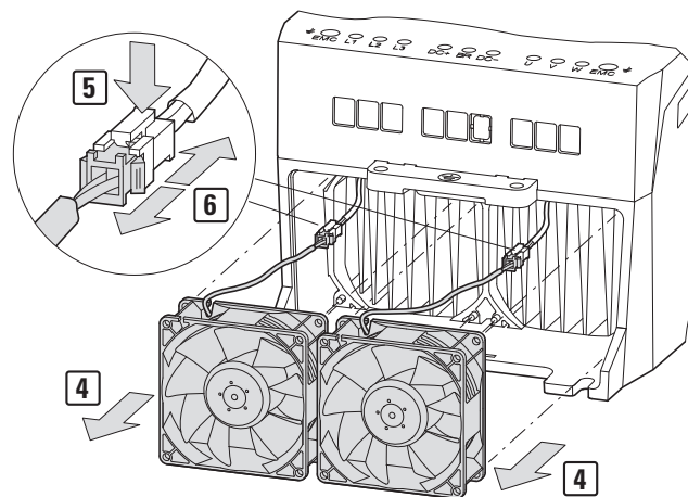
Figure 26: Remove fan
