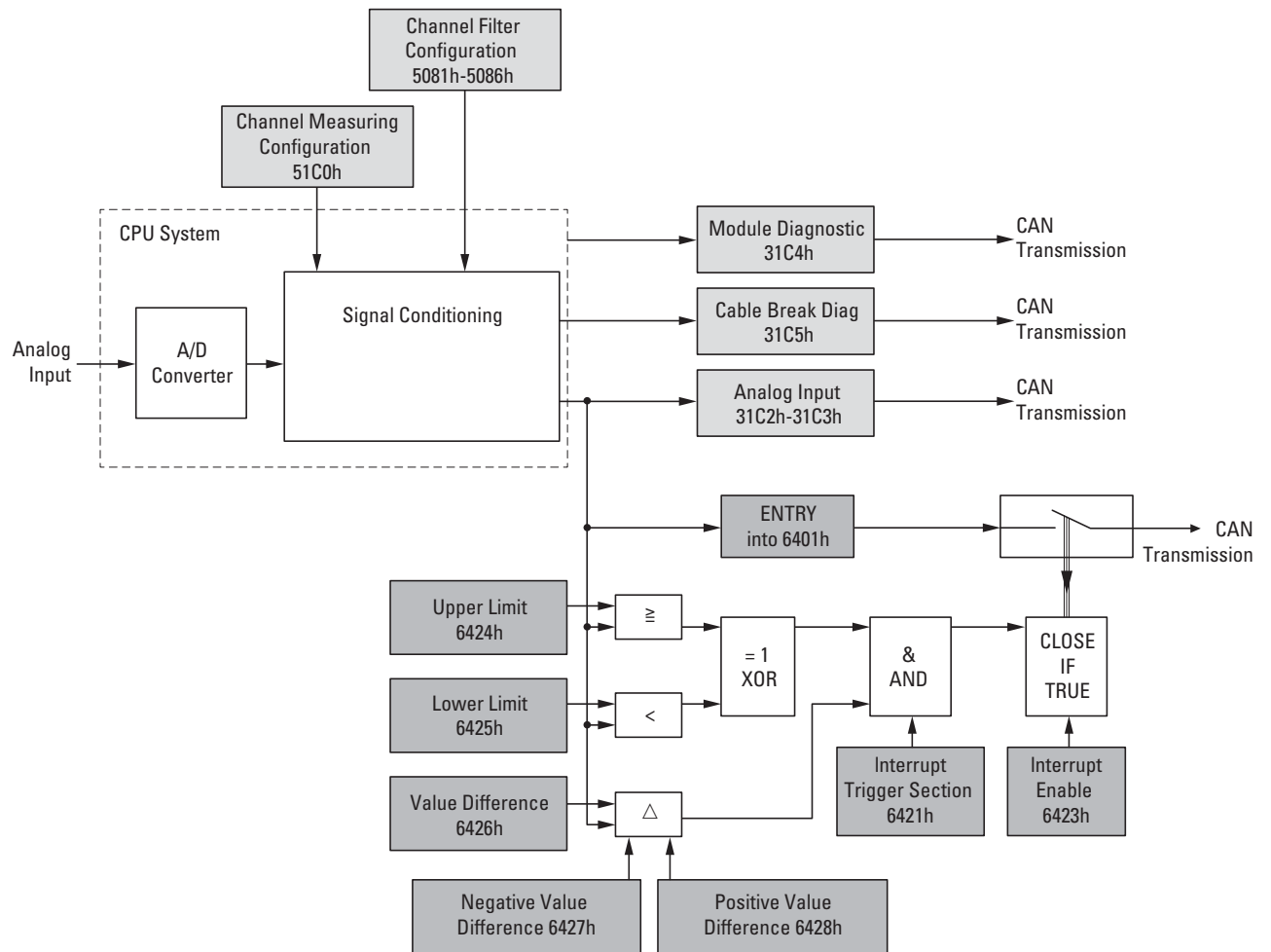
Abbildung 73: Blockschaltbild der verschiedenen CANopen Objekte zur Übertragung von Datenströme
