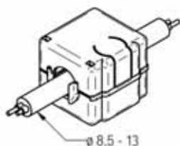
Abbildung 27: Abschirmen mit Einrastferrithülse
