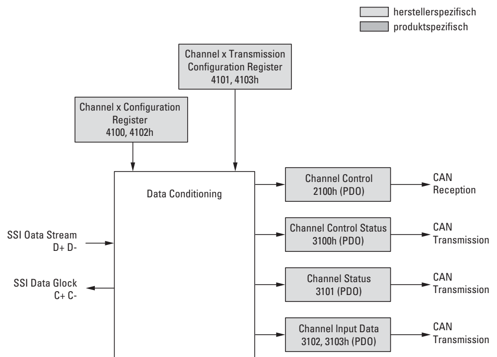
Abbildung 94: Blockschaltbild der verschiedenen CANopen Objekte zur Übertragung von Datenströme
