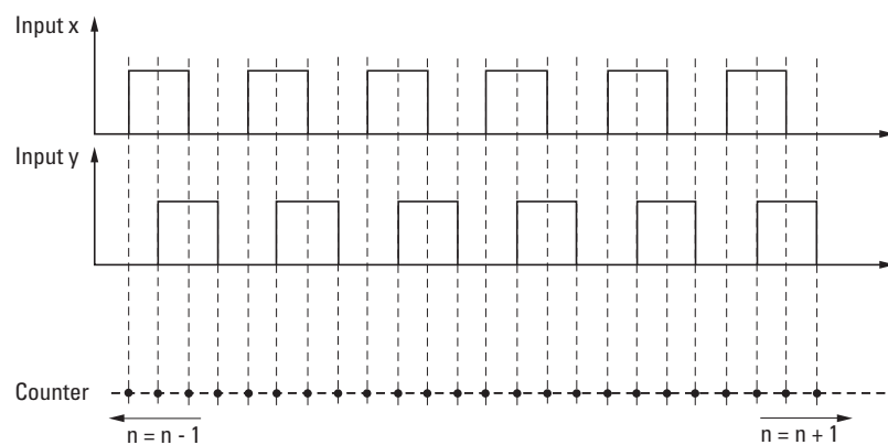
Abbildung 70: Zählweise an den Eingängen (x/y) = (1/2) oder (3/4) des Incremental Encoder Registers von XN-322-16DIO-PC05 mit Counter 4-fach Auswertung
