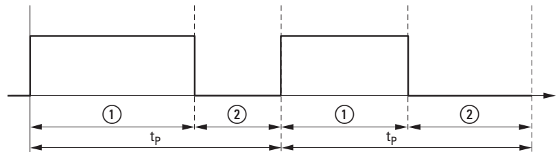
Abbildung 71: PWM Signalmessung
