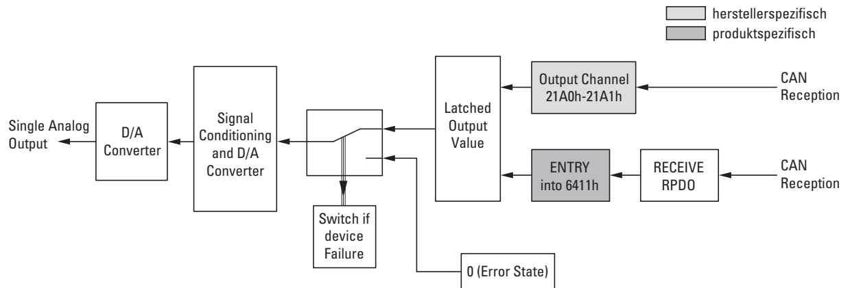
Abbildung 82: Blockschaltbild der verschiedenen CANopen Objekte für analoge Ausgänge
