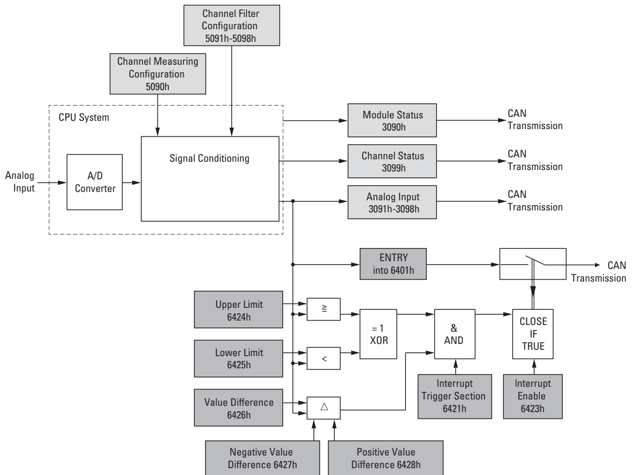
Abbildung 76: Blockschaltbild der verschiedenen CANopen Objekte für analoge Eingänge
