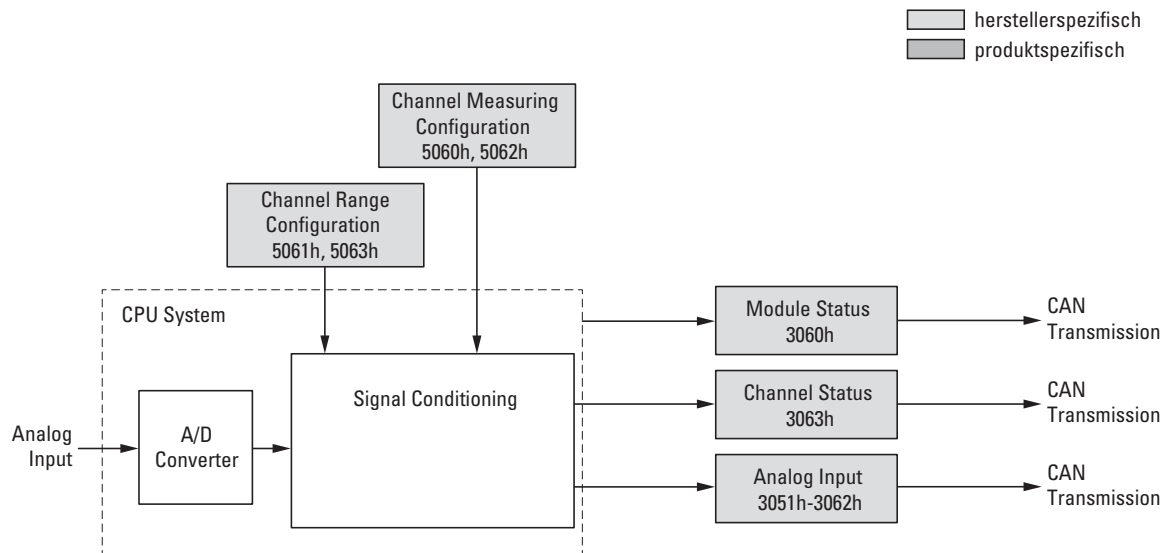
Abbildung 89: Blockschaltbild der verschiedenen CANopen Objekte
