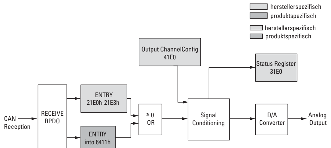
Abbildung 79: Blockschaltbild der verschiedenen CANopen Objekte zur Übertragung von Datenströme
