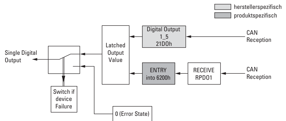
Abbildung 60: Blockschaltbild der verschiedenen CANopen Objekte zur Übertragung von Datenströme
