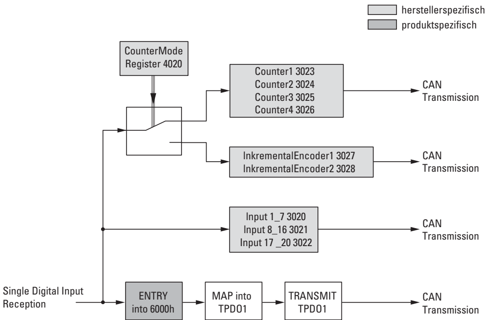
Abbildung 56: Blockschaltbild der verschiedenen CANopen Objekte für digitale Eingänge
