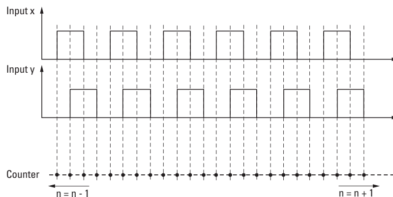
Abbildung 57: Zählweise an den Eingängen des Incremental Encoder Registers von XN-322-20DI-PCNT mit Counter 4-fach Auswertung
