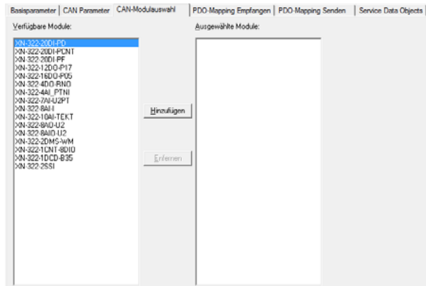
Abbildung 36: CAN Modulauswahl des CAN-Slaves (hier: XN-312-GW-CAN)
