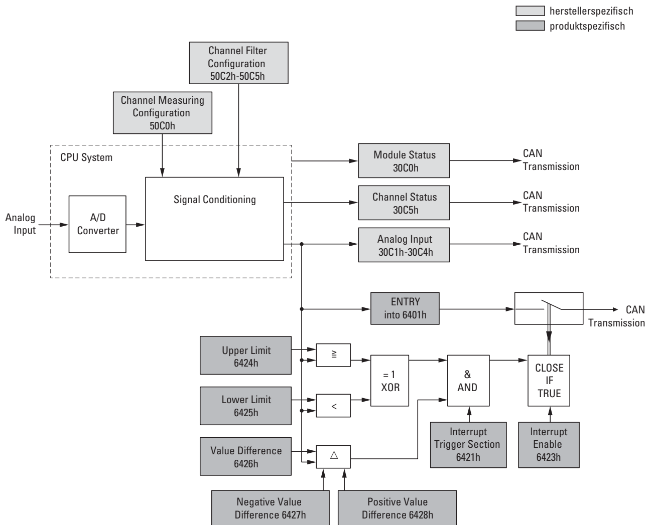
Abbildung 87: Blockschaltbild der verschiedenen CANopen Objekte für analoge Eingänge
