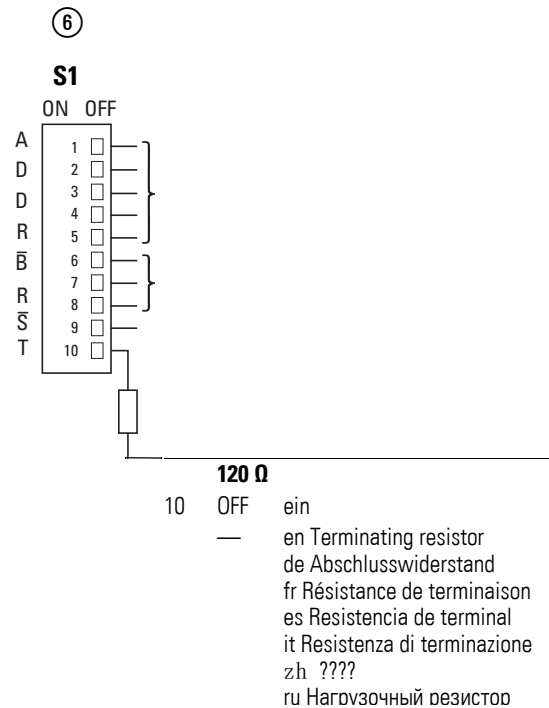
Abbildung 7: DIP-Schalter zur Aktivierung des Abschlusswiderstands
