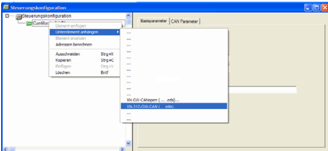
Abbildung 34: CAN-Slave anhängen
