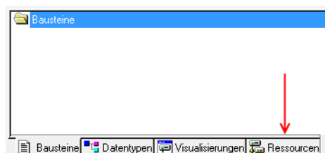
Abbildung 31: Konfigurationsmodus anwählen
