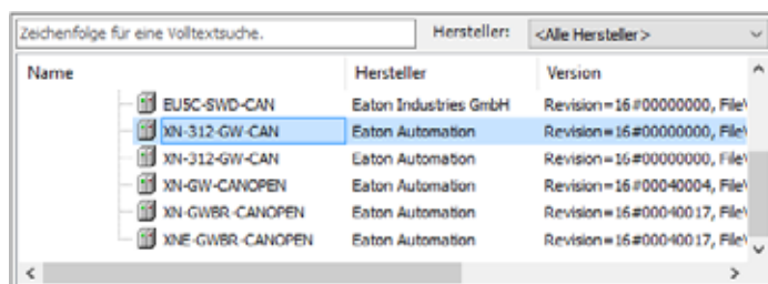
Abbildung 44: CANopen-Device anhängen
