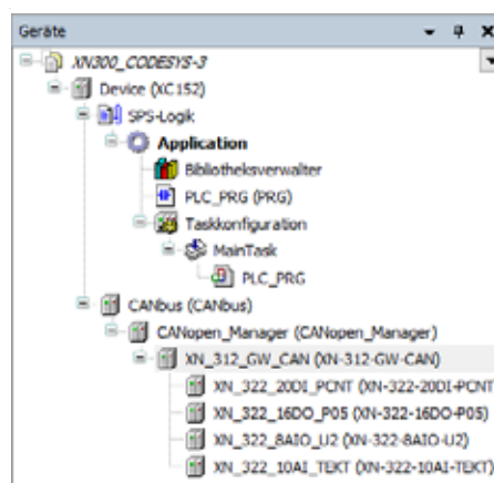
Abbildung 46: Konfigurationsbaum „Geräte“
