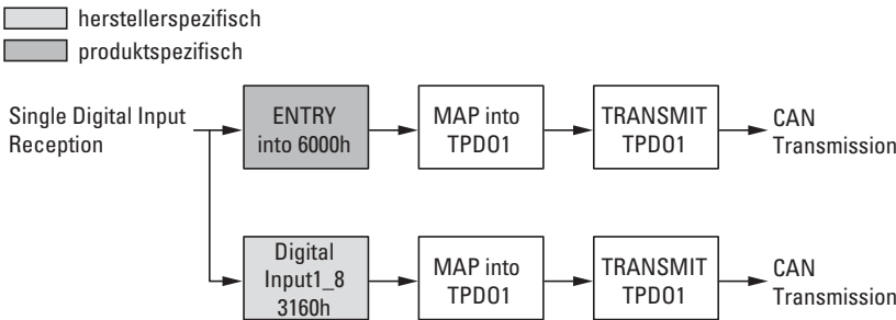
Abbildung 66: Blockschaltbild der verschiedenen CANopen Objekte für digitale Eingänge
