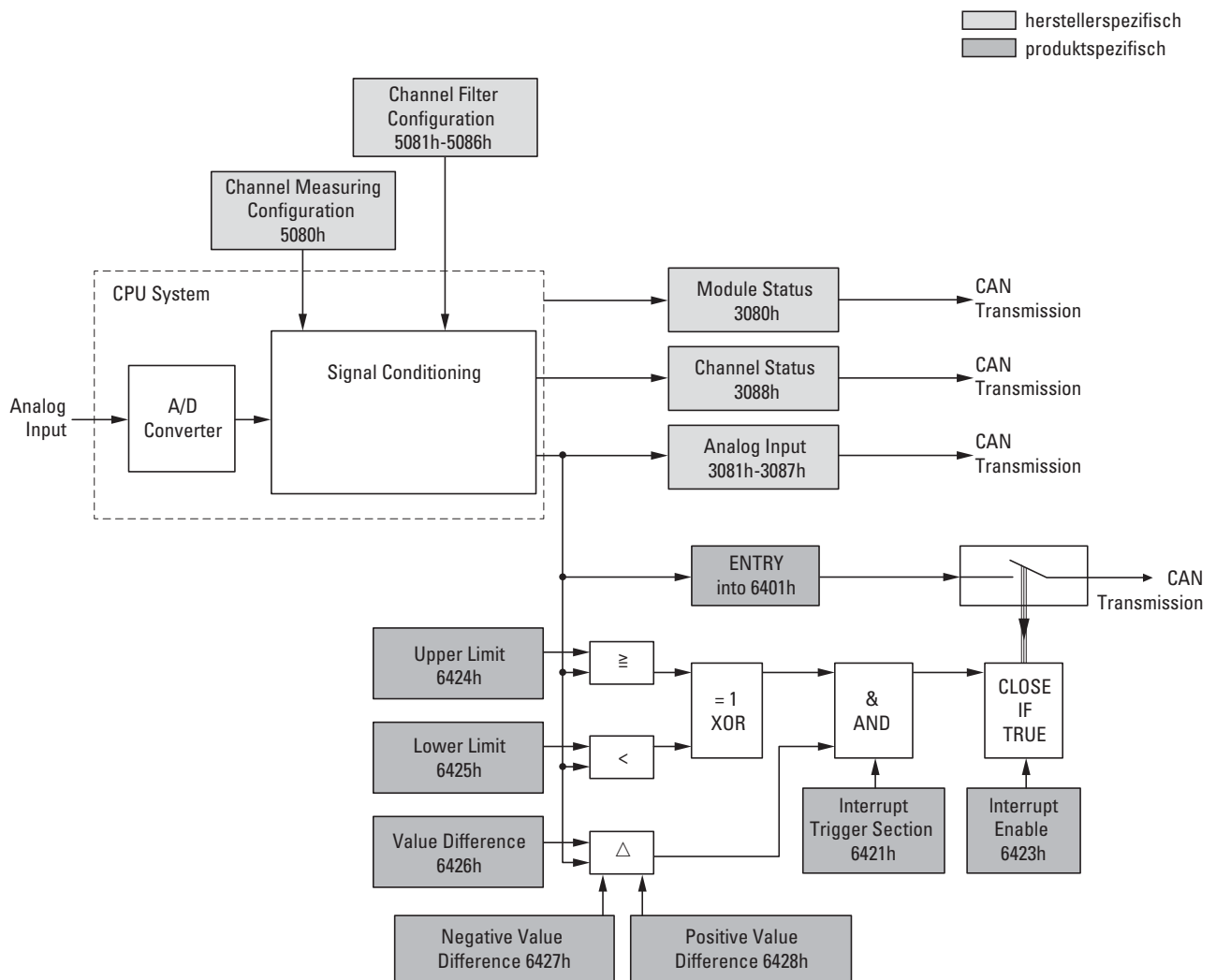
Abbildung 75: Blockschaltbild der verschiedenen CANopen Objekte für analoge Eingänge
