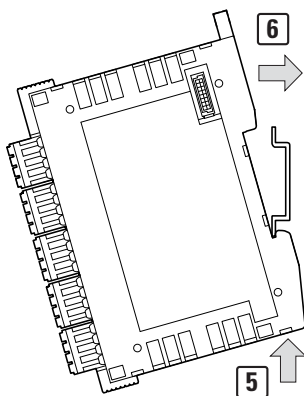
Abbildung 14: Systemblock an Unterkante Hutschiene ansetzen
