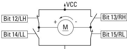
Prinzipschaltbild Motordrehrichtung links
