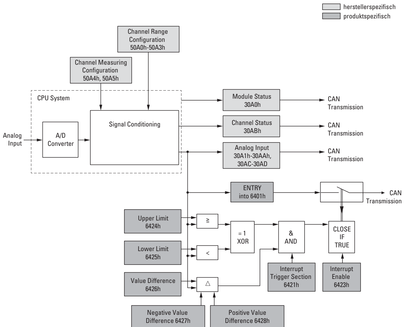
Abbildung 78: Blockschaltbild der verschiedenen CANopen Objekte
