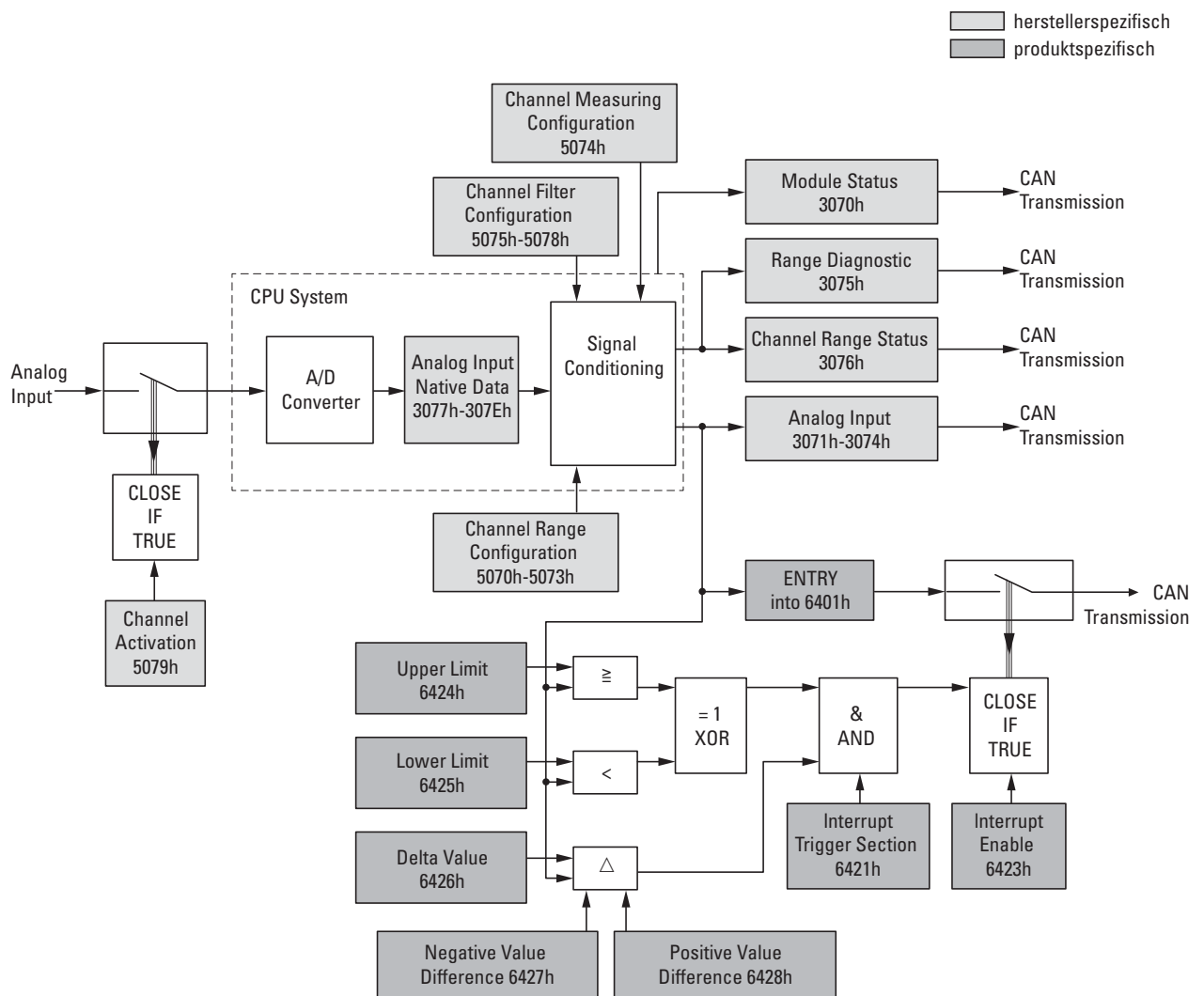
Abbildung 74: Blockschaltbild der verschiedenen CANopen Objekte für analoge Eingänge
