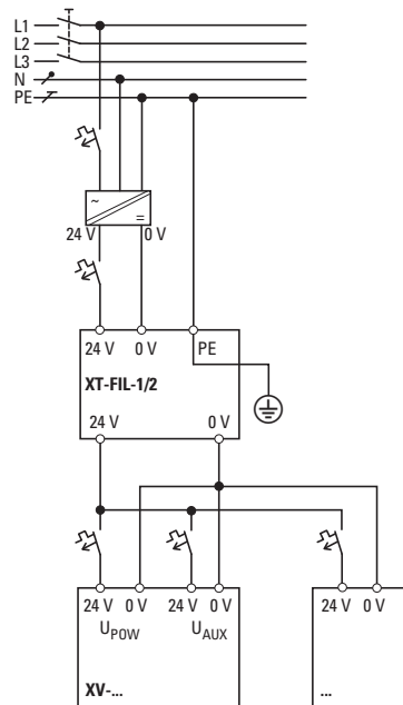
Abbildung 26: Projektierungsbeispiel zur Integration der Entstörfilter
