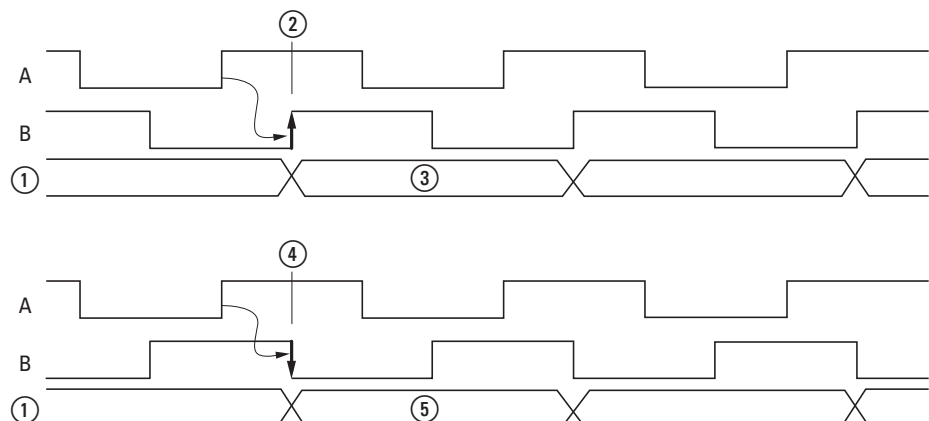
Abbildung 92: Wirkdiagramm Signale A, B
