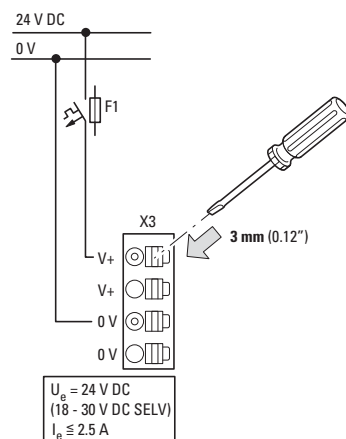
Abbildung 21: Anschluß der Spannungsversorgung
