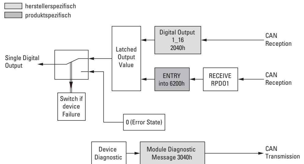
Abbildung 62: Blockschaltbild der verschiedenen CANopen Objekte für digitale Ausgänge
