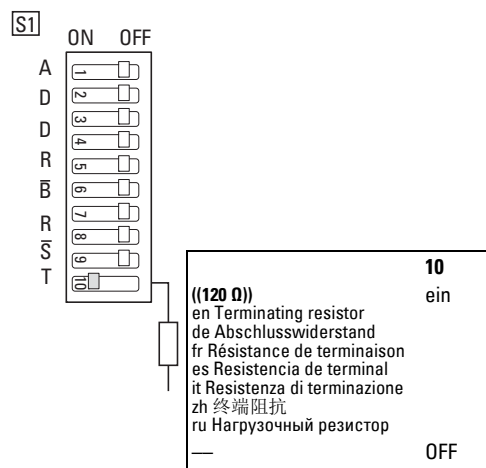
Abbildung 9: Abschlusswiderstand aktiviert
