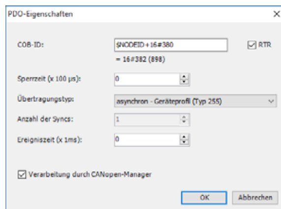
Abbildung 49: Übertragungstyp des manuell gemappten PDOs festlegen
