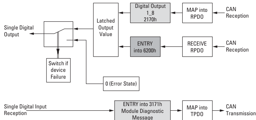
Abbildung 69: Blockschaltbild der verschiedenen CANopen Objekte für digitale Ausgänge
