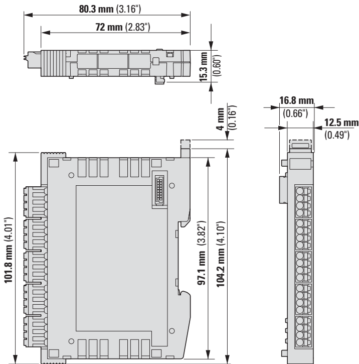
Abbildung 103: Abmessungen XN-312-GW-CAN
