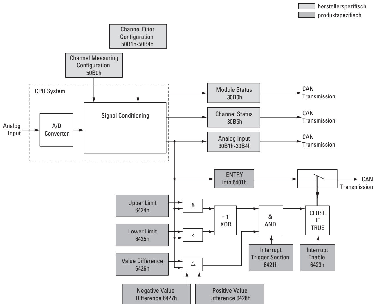
Abbildung 83: Blockschaltbild der verschiedenen CANopen Objekte für analoge Eingänge
