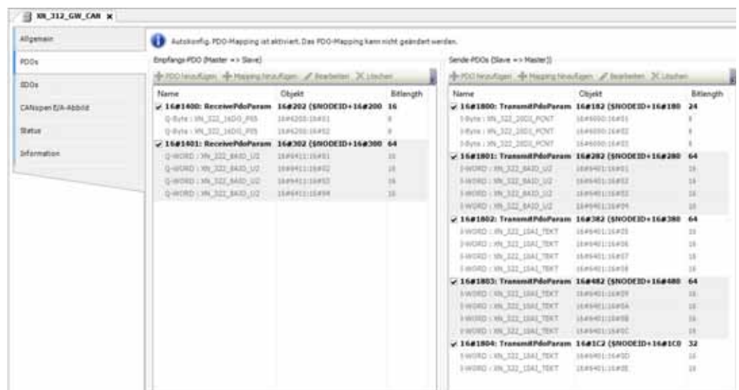
Abbildung 48: Mappingtabelle Registerkarte „PDOs (Process Data Object)“
