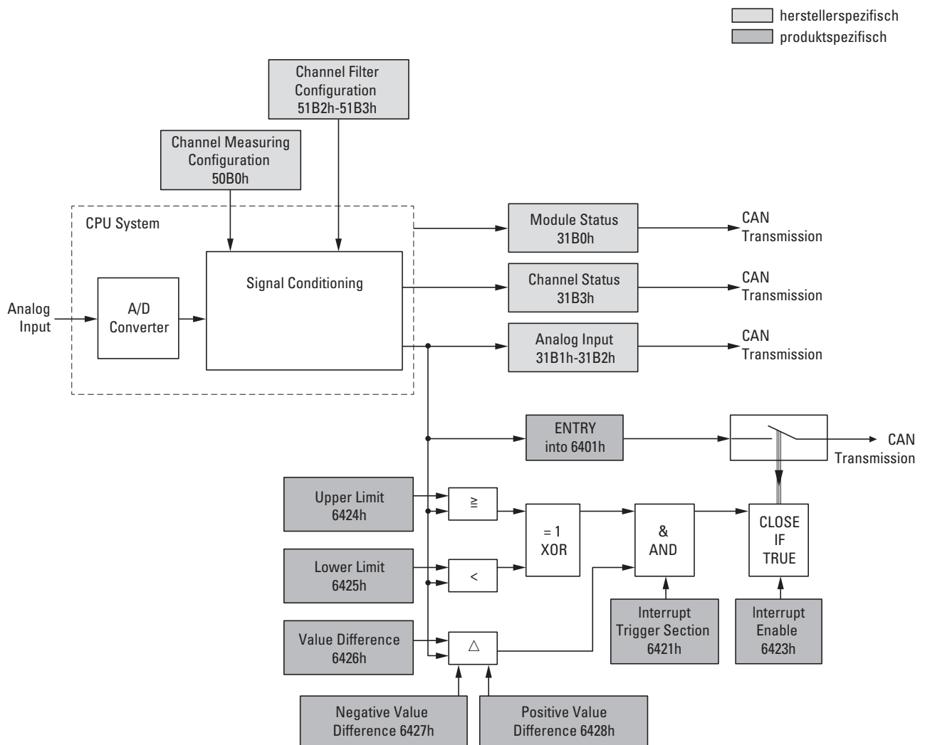
Abbildung 85: Blockschaltbild der verschiedenen CANopen Objekte für analoge Eingänge
