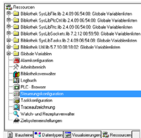
Abbildung 32: Steuerungskonfiguration anwählen
