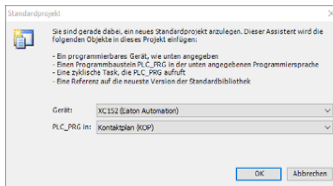
Abbildung 38: Standardprojekt einstellen
