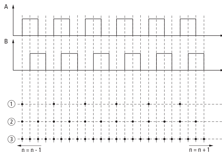
Abbildung 93: Wirkdiagramm
