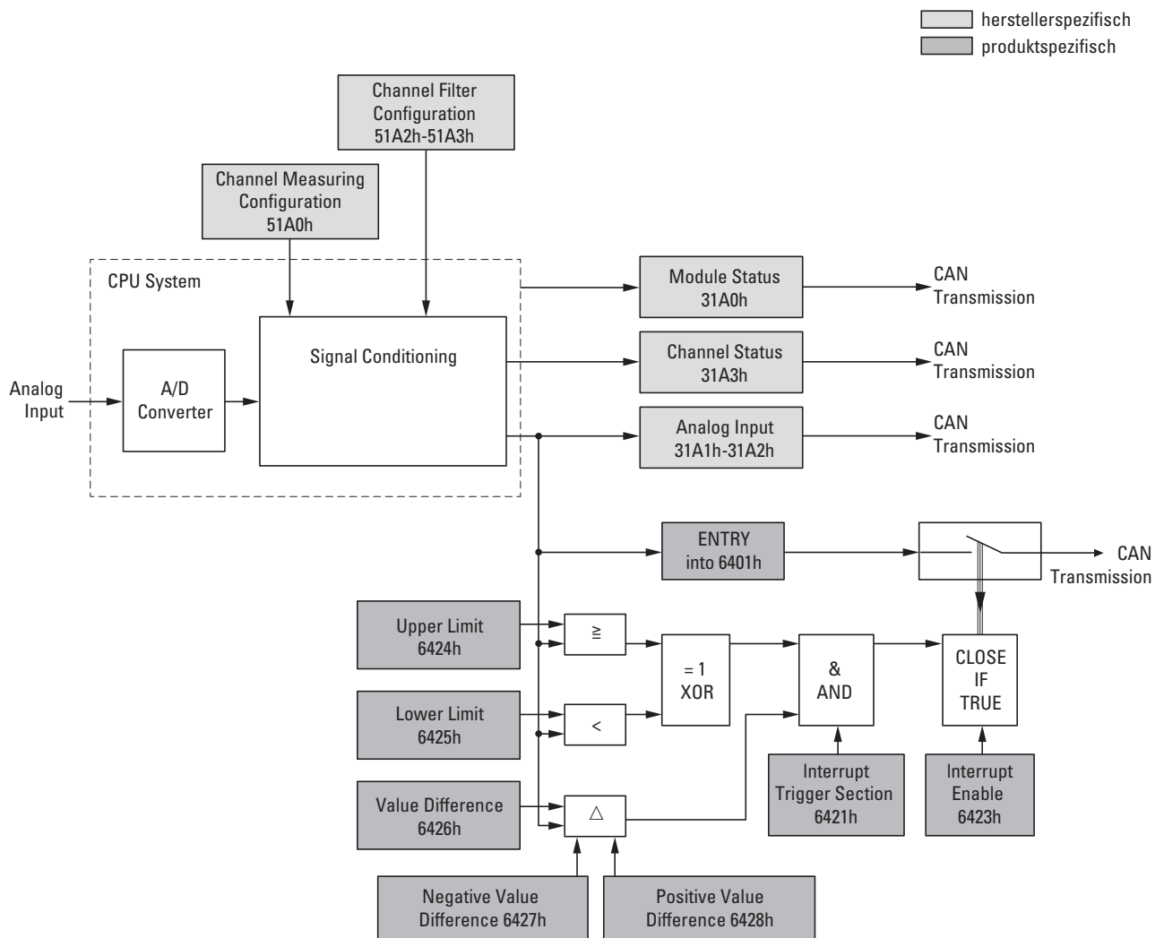
Abbildung 81: Blockschaubild der verschiedenen CANopen Objekte für analoge Eingänge
