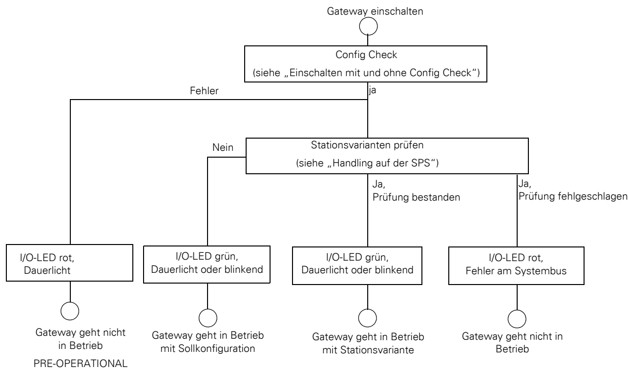
Abbildung 100:Mögliche Betriebsarten des Gateways
