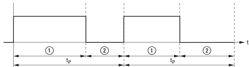
Abbildung 72: PWM Signalmessung ① High Time ② Low Time
