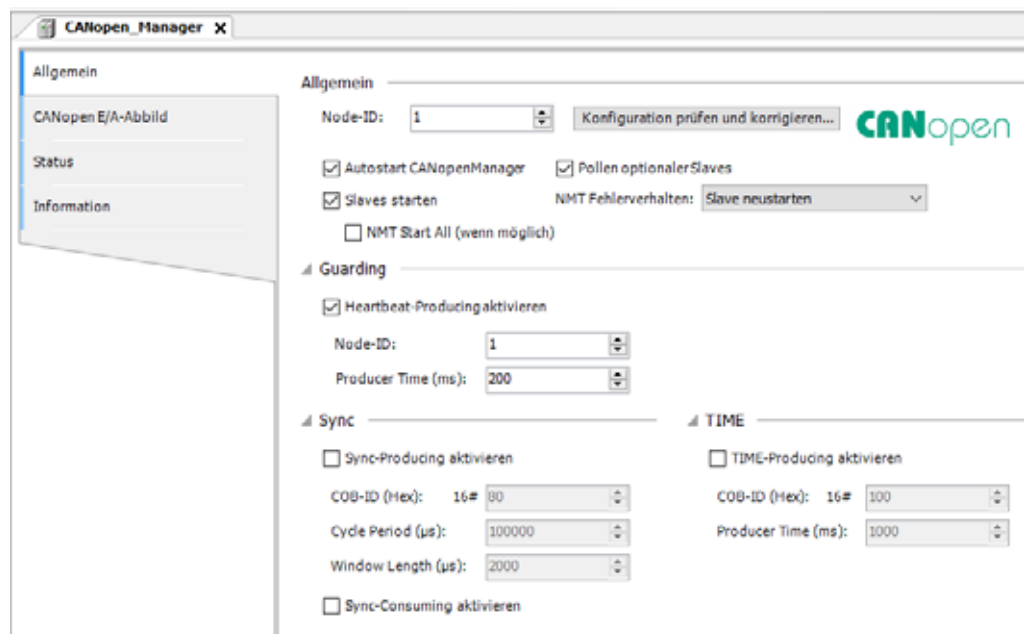
Abbildung 42: CAN Parameter des CANopen Managers
