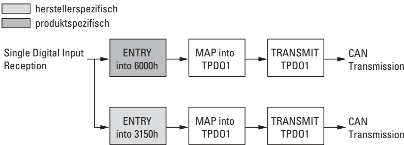
Abbildung 52: Blockschaltbild der verschiedenen CANopen Objekte für digitale Eingänge
