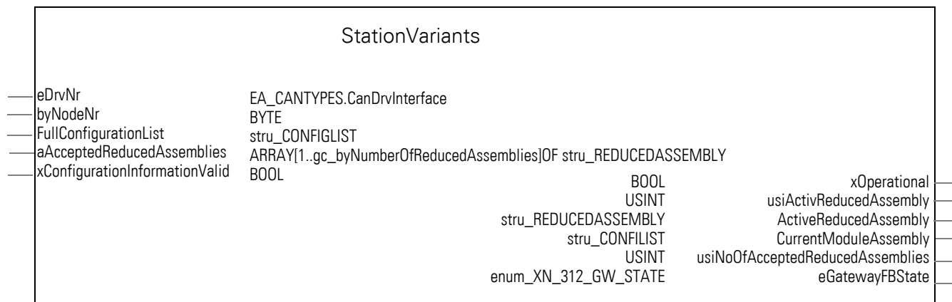
Abbildung 99: Funktionsbaustein StationVariants der Bibliothek EA_XN300
