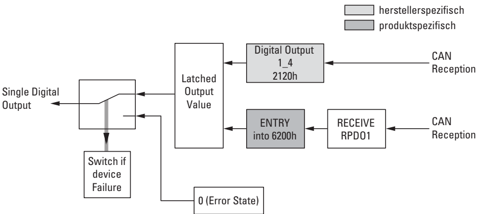
Abbildung 59: Blockschaltbild der verschiedenen CANopen Objekte für digitale Ausgänge
