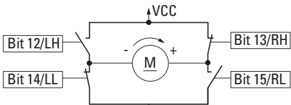
Prinzipschaltbild Motordrehrichtung rechts
