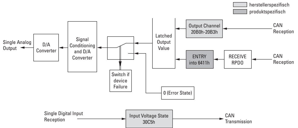
Abbildung 88: Blockschaltbild der verschiedenen CANopen Objekte für analoge Ausgänge
