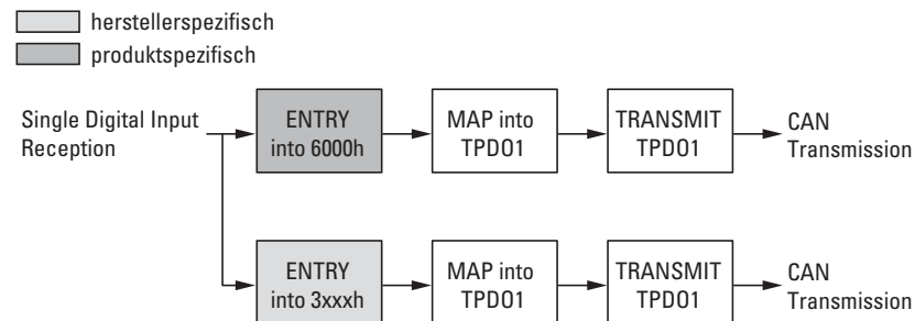
Abbildung 58: Blockschaltbild der verschiedenen CANopen Objekte für digitale Eingänge
