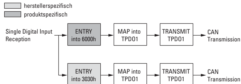
Abbildung 55: Blockschaltbild der verschiedenen CANopen Objekte für digitale Eingänge
