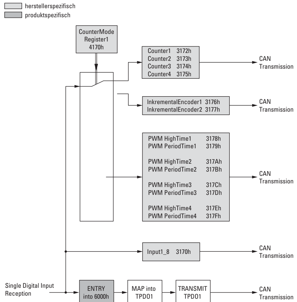
Abbildung 68: Blockschaltbild der verschiedenen CANopen Objekte für digitale Eingänge
