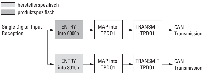
Abbildung 54: Blockschaltbild der verschiedenen CANopen Objekte für digitale Eingänge
