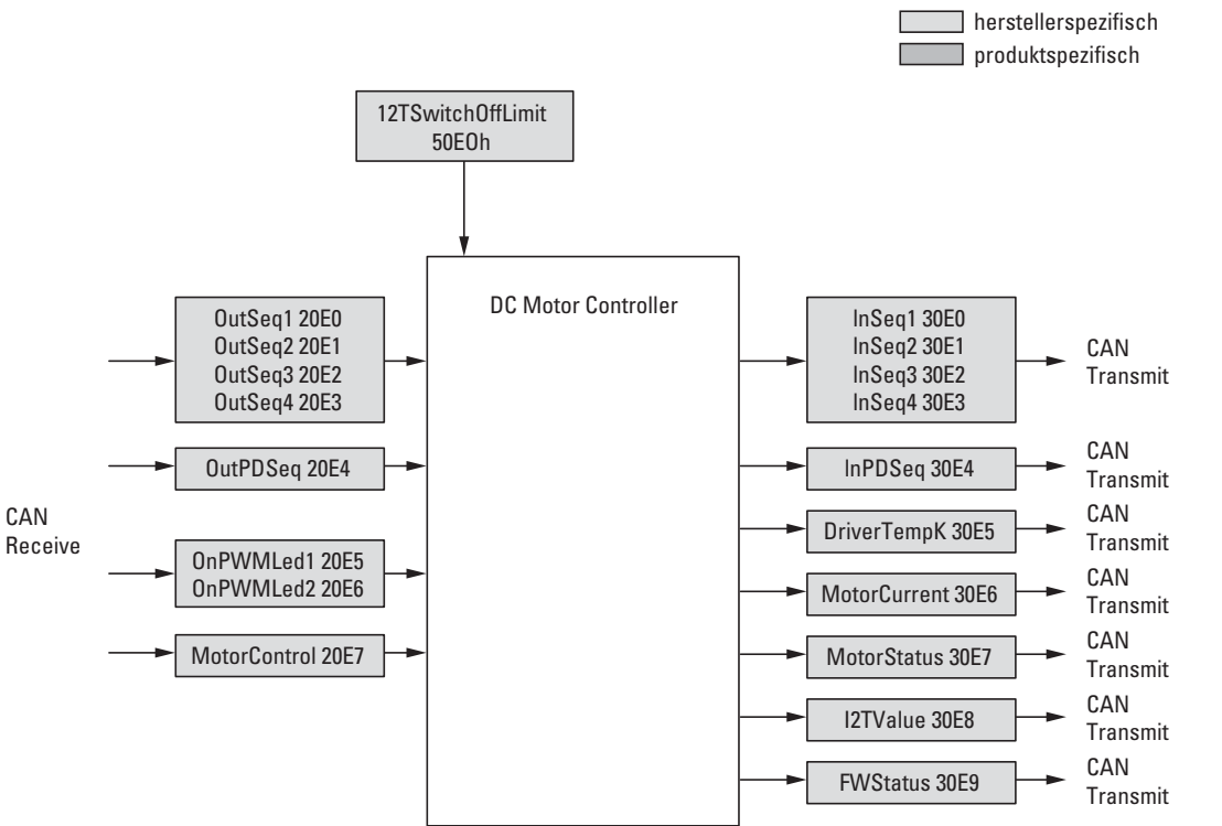
Abbildung 90: Blockschaltbild der verschiedenen CANopen Objekte
