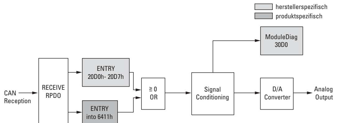
Abbildung 80: Blockschaltbild der verschiedenen CANopen Objekte für analoge Ausgänge
