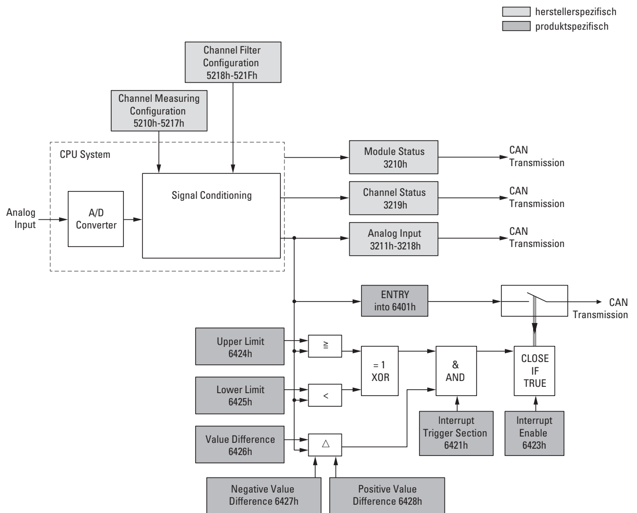
Abbildung 77: Blockschaftbild der verschiedenen CANopen Objekte zur Übertragung von Datenströme
