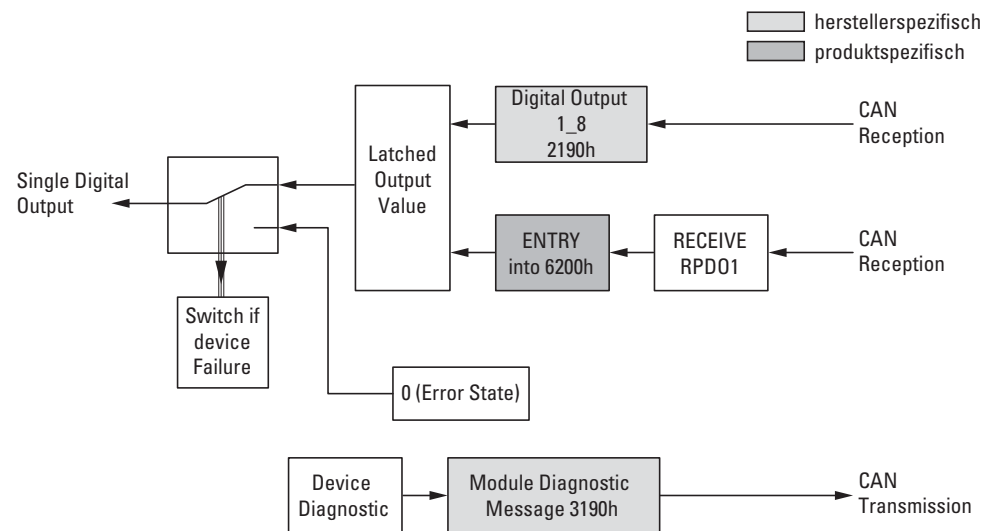
Abbildung 61: Blockschaubild der verschiedenen CANopen Objekte für digitale Ausgänge
