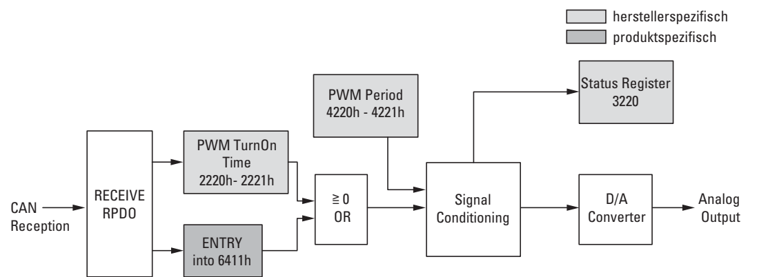
Abbildung 95: Blockschaltbild der verschiedenen CANopen Objekte zur Übertragung von Datenströme
