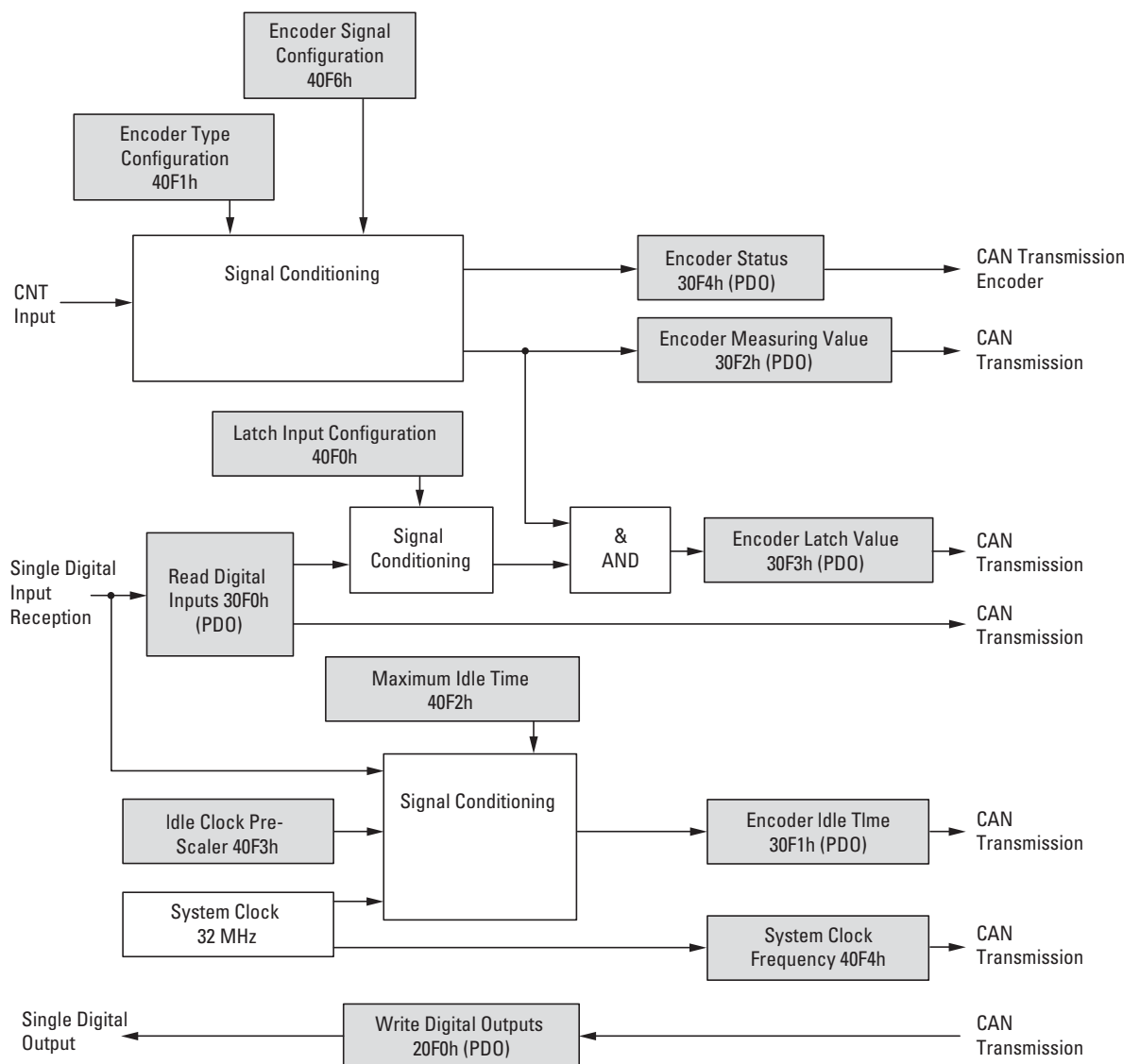
Abbildung 91: Blockschaltbild der verschiedenen CANopen Objekte für analoge Eingänge
