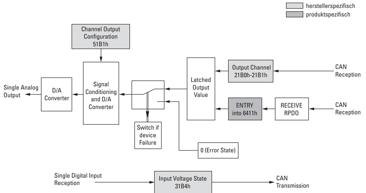
Abbildung 86: Blockschaltbild der verschiedenen CANopen Objekte für analoge Ausgänge
