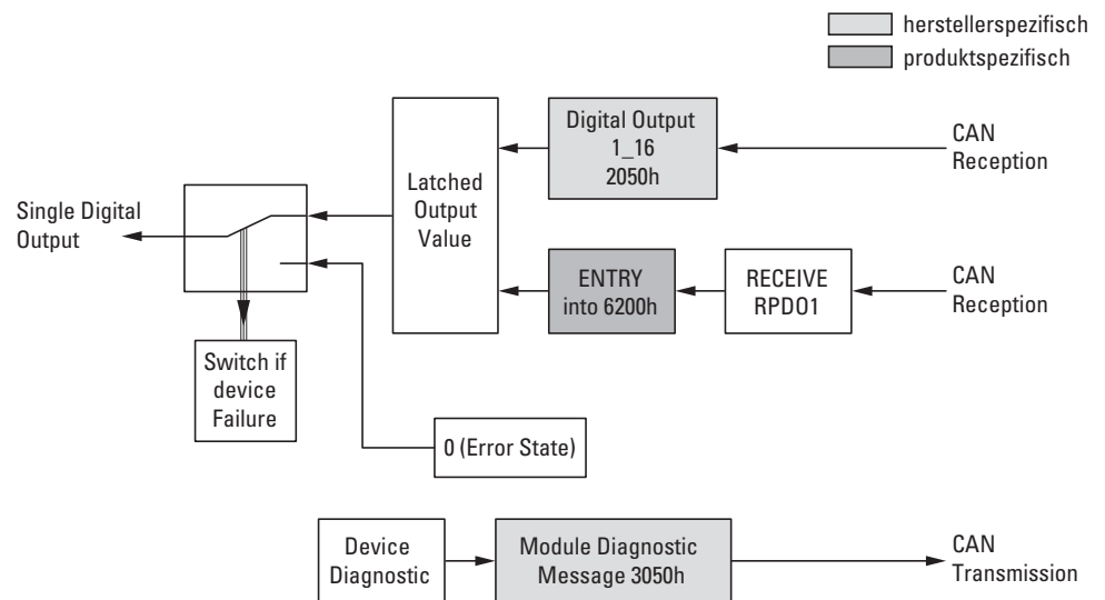
Abbildung 63: Blockschaltbild der verschiedenen CANopen Objekte für digitale Ausgänge
