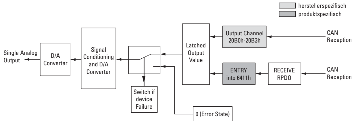
Abbildung 84: Blockschaltbild der verschiedenen CANopen Objekte für analoge Ausgänge
