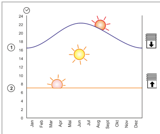
Abb. 29: Anwendungsbeispiel Jalousiesteuerung 1
