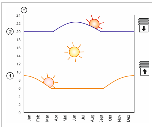
Abb. 31: Anwendungsbeispiel Jalousiesteuerung 3
