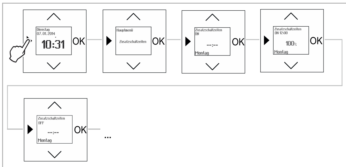
Abb. 22: Menüpunkt - Zusatzschaltzeiten Licht
