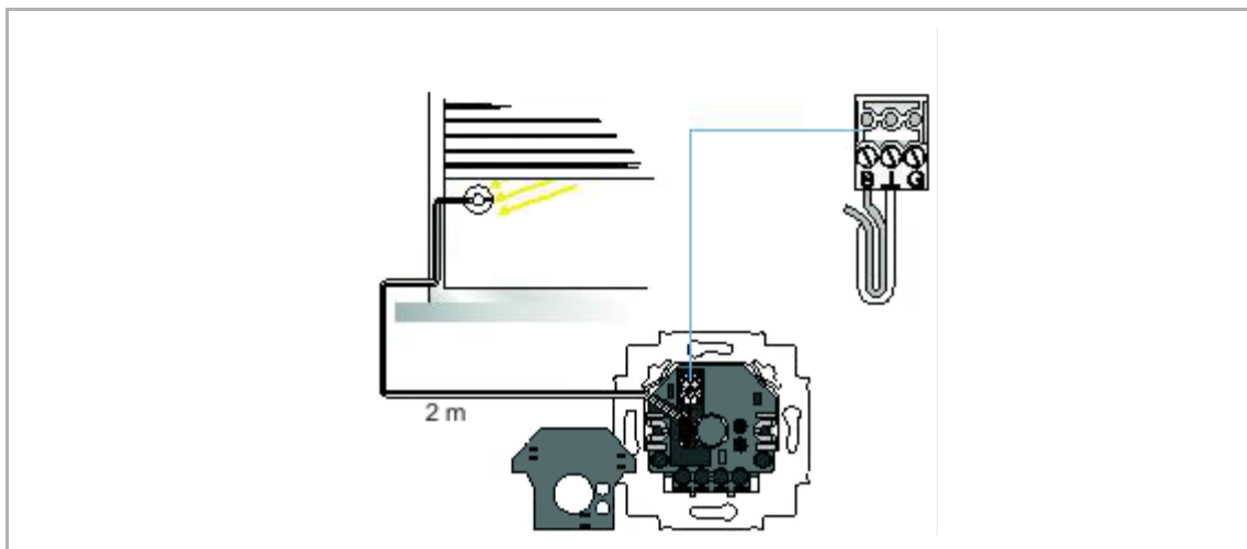
Abb. 1: Angeschlossener Helligkeitssensor: Der Sensor kann an beliebiger Stelle auf der Scheibe angebracht werden
