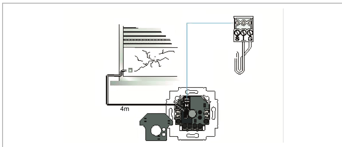
Abb. 2: Angeschlossener Glasbruchmelder
