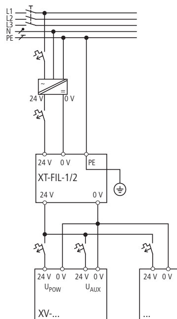
Abb. 17: Projektierungsbeispiel zur Integration der Entstörfilter
