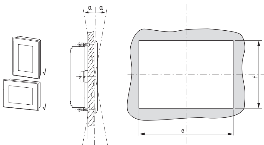
Abb. 16: Einbaulage
