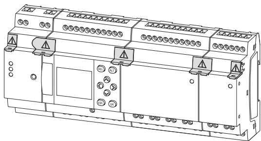
Fig. 343: Ejemplo de módulo de control easyE4 con ampliaciones de E/S y módulo de comunicación easy EASY-COM-SWD-...
