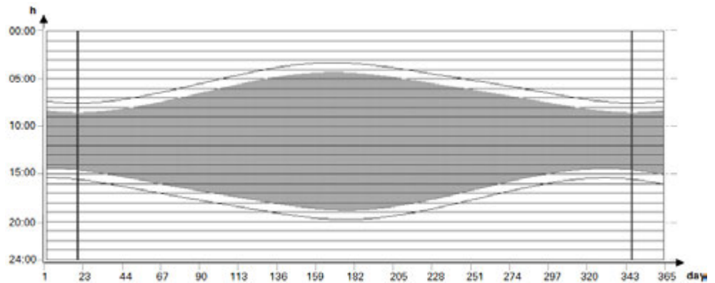
Fig. 167: Offset O1=1; O2= -1; Q1=1 se conecta 1 hora tras la salida del sol y 1 hora antes de la puesta del sol
