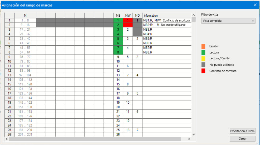
Fig. 125: Asignación del rango de marcas con conflicto de escritura en MW1
