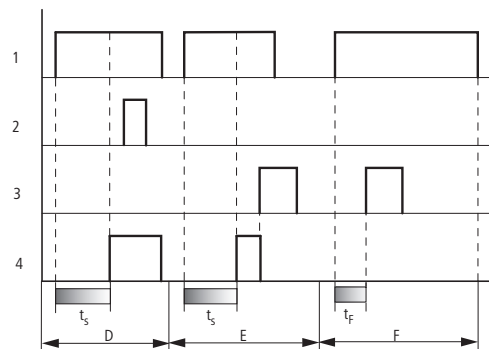
Fig. 146: Diagrama de comportamiento relé temporizador con temporización de trabajo (con/sin conexión aleatoria)
