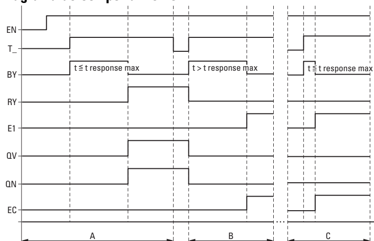
Fig. 252: Diagrama de comportamiento contador de frecuencia
