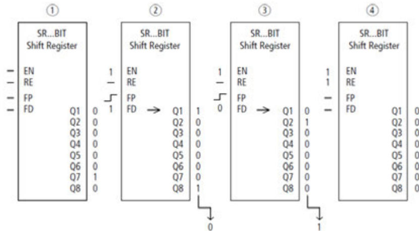
Fig. 219: Registro de desplazamiento SR...: operación hacia delante en el modo de funcionamiento BIT
