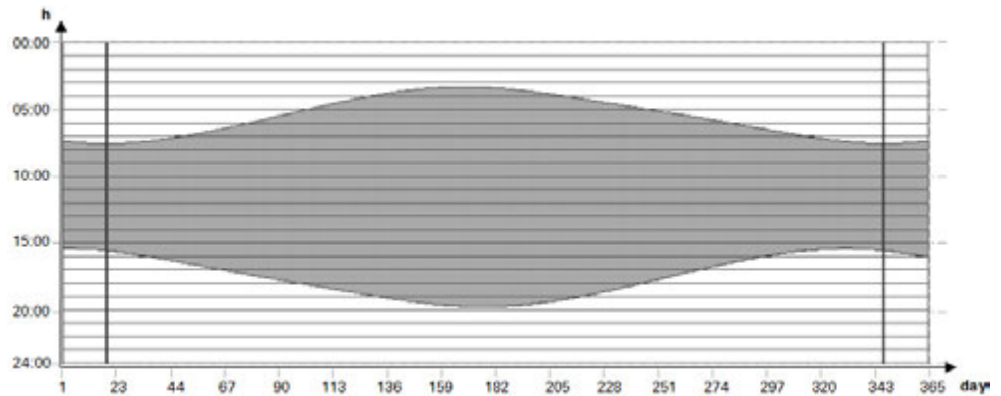
Fig. 166: Sin offset; O1=0; O2=0; Q1=1 entre la salida y la puesta del sol
