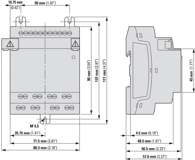
Fig. 399: Dimensiones en mm (pulgadas) ampliaciones 4 ud. división
