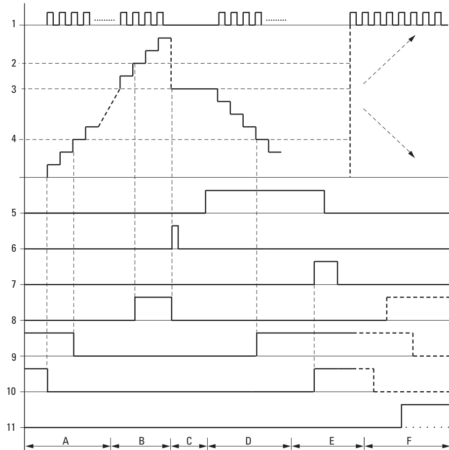
Fig. 172: Diagrama de comportamiento Relé contador
