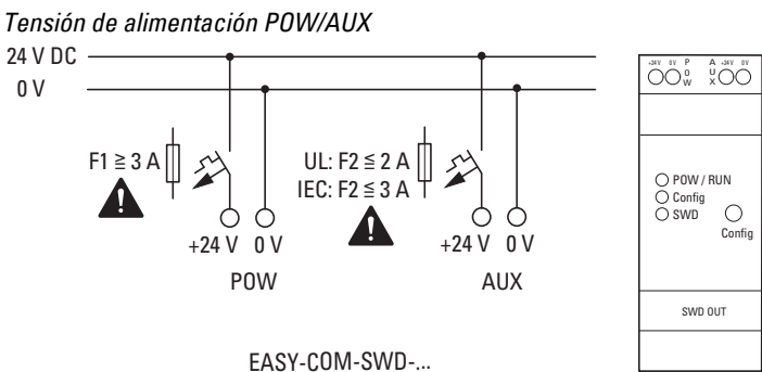
Fig. 345: Conectar la tensión de alimentación EASY-COM-SWD-...
