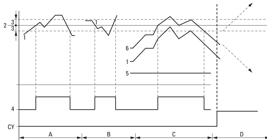
Fig. 178: Diagrama de comportamiento comparador de valores analógicos
