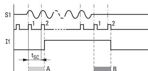
Fig. 310: Comportamiento de conexión de la señal de entrada AC con la función contra rebotes I activada
