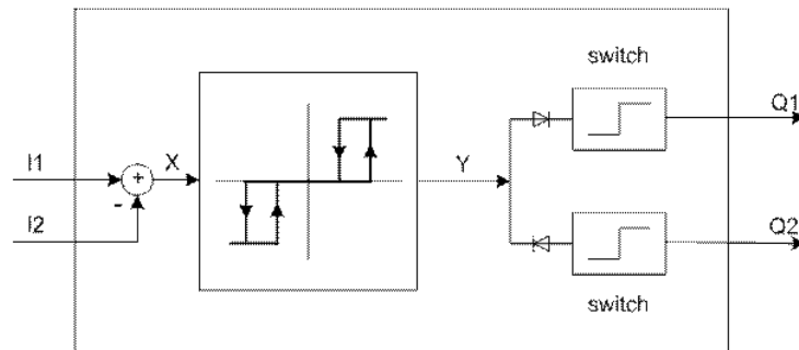
Fig. 203: Esquema de contactos básico Regulador de tres vías
