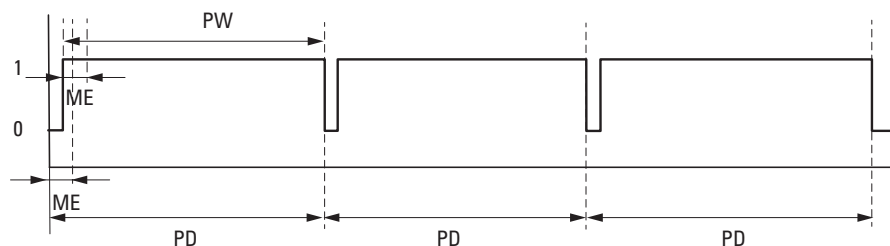
Fig. 191: En la salida del módulo se muestra la señal continua con SV = 3768, ME = 93 ms, PD=1000 ms; E1 = 1
