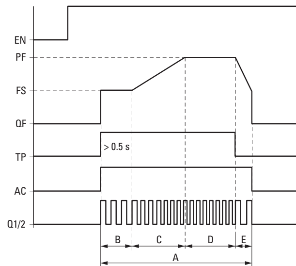
Fig. 201: Diagrama de comportamiento Modo desplazamiento con frecuencia de impulso determinada, P1 alcanzado tras la fase de frenado
