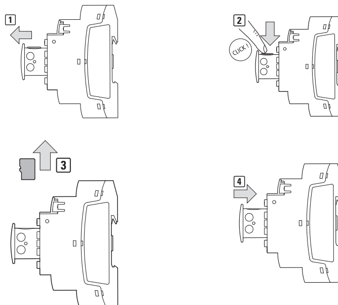
Fig. 35: Retirar la tarjeta de memoria
