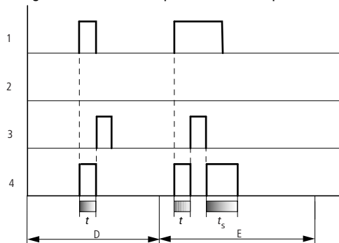
Fig. 151: Diagrama de comportamiento relé temporizador, generación de un impulso a partir de una señal 2
