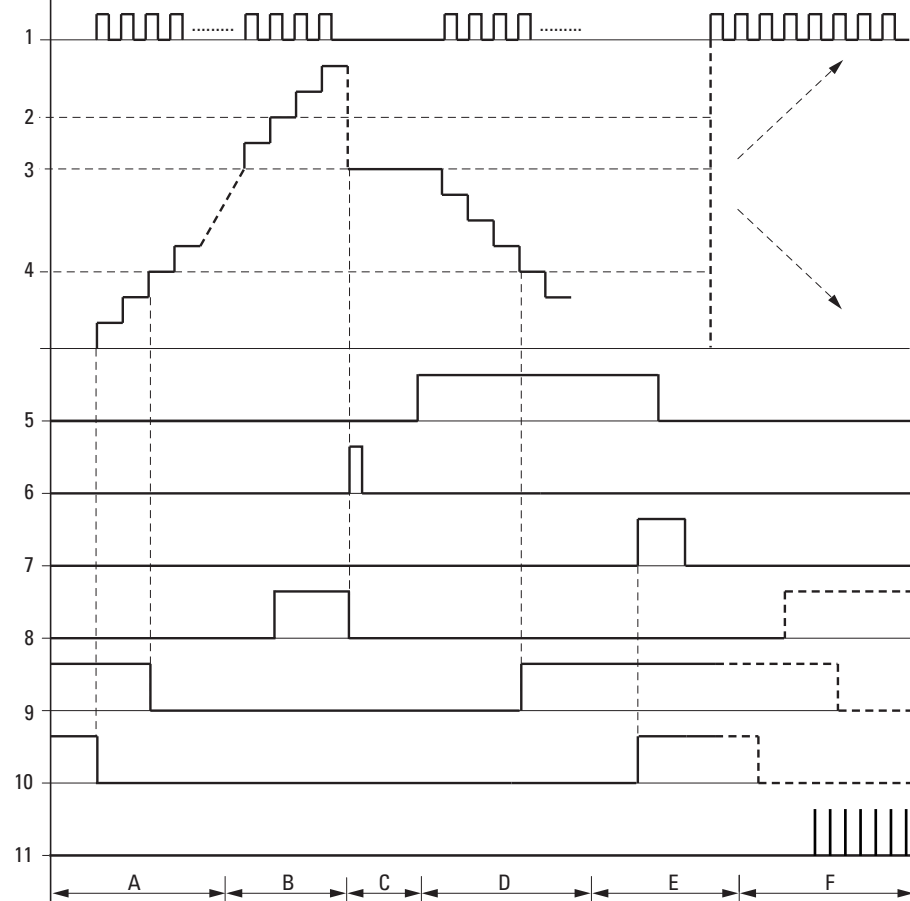
Fig. 177: Diagrama de comportamiento Contador incremental rápido
