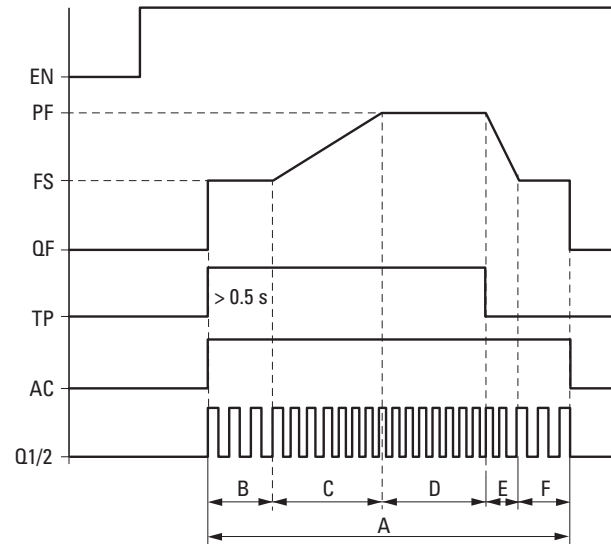
Fig. 202: Diagrama de comportamiento Modo desplazamiento con frecuencia de impulso pre-determinada, P1 no alcanzado tras la fase de frenado
