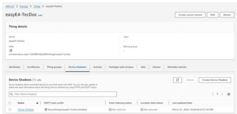
Fig. 356: Ejemplo: AWS-Register Device Shadows
