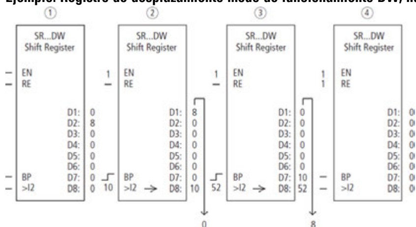
Fig. 220: Registro de desplazamiento SR.: operación hacia atrás en el modo de funcionamiento DW
