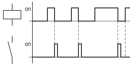
Fig. 103: Diagrama de comportamiento "impulso de ciclo" con flanco negativo
