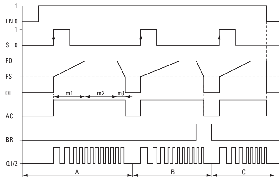
Fig. 199: Diagrama de comportamiento salida de impulso PO con número de impulsos predeterminado I1 - posibles fases del funcionamiento normal
