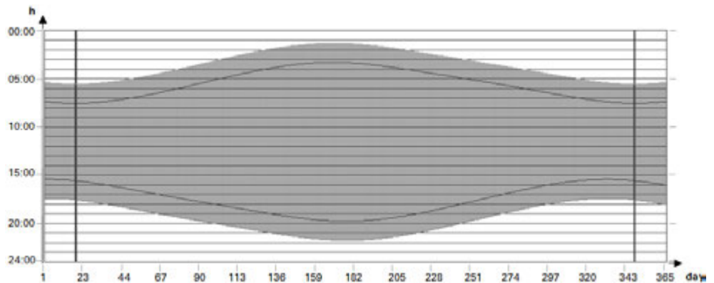
Fig. 168: Offset; O1=-2; O2=2; Q1=1 se conecta 2 horas antes de la salida del sol y 2 horas tras la puesta del sol
