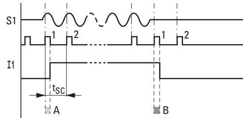
Fig. 311: Comportamiento de conexión de la señal de entrada AC con la función contra rebotes I desactivada
