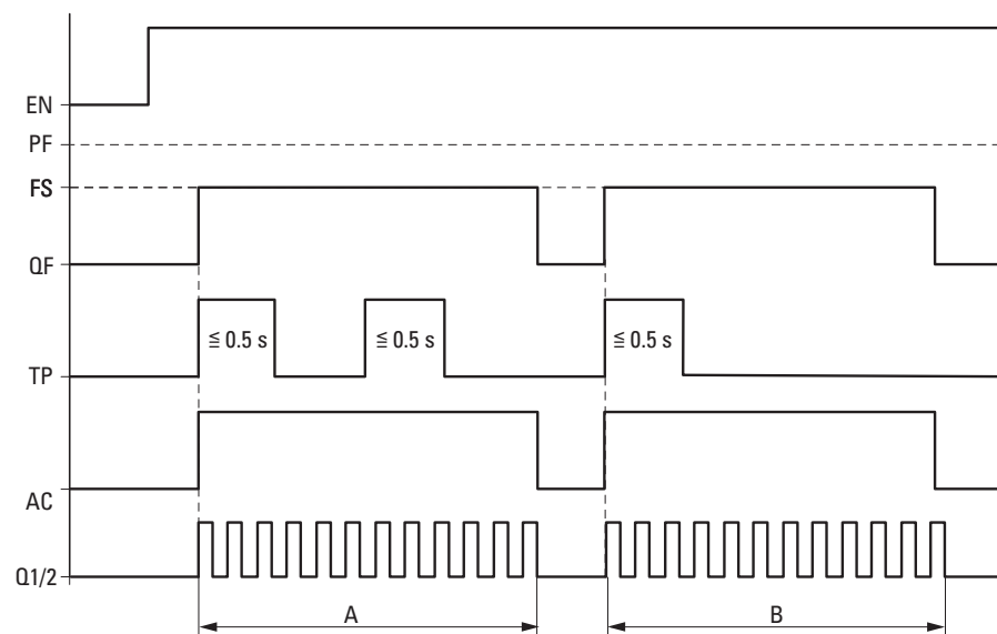
Fig. 200: Diagrama de comportamiento Modo desplazamiento con número de pasos predeterminado P1
