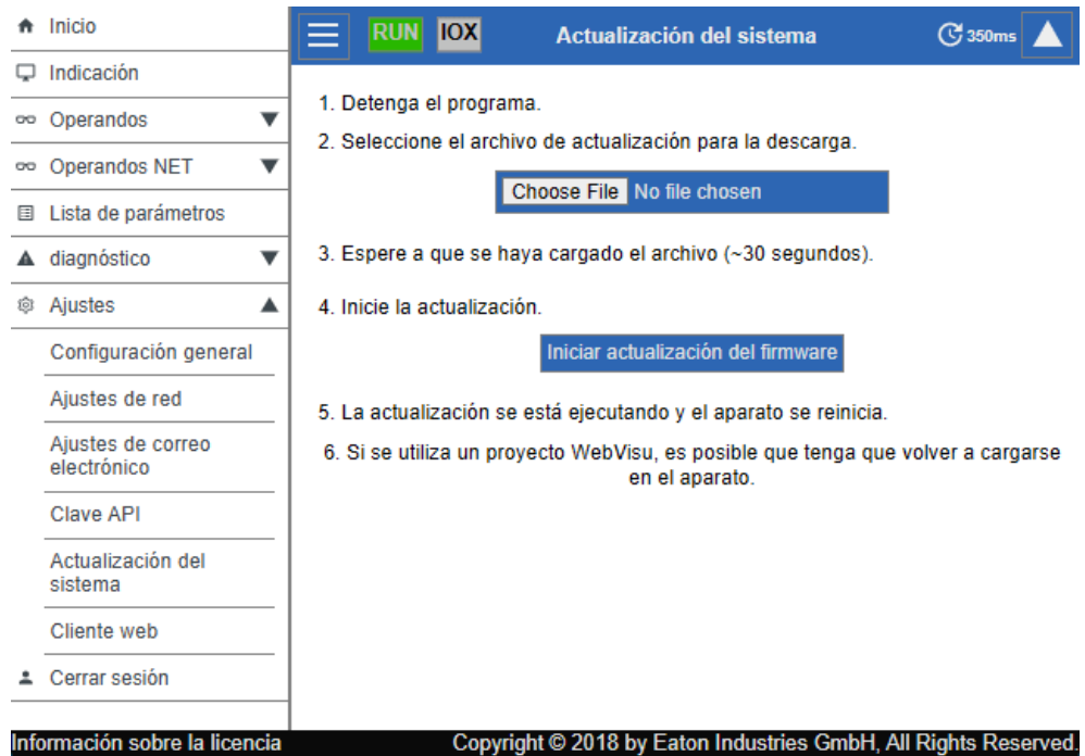
Fig. 335: Web-Client, actualización del sistema
