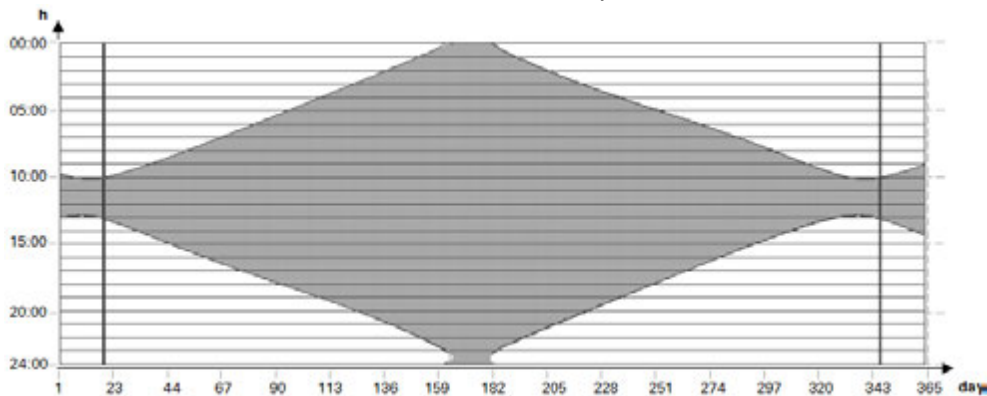
Fig. 164: Salida y puesta del sol en Drevja
