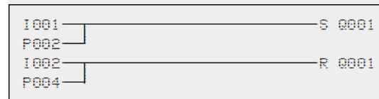
Fig. 114: Conectar Q1 mediante I1, I2, Í, o Ú
