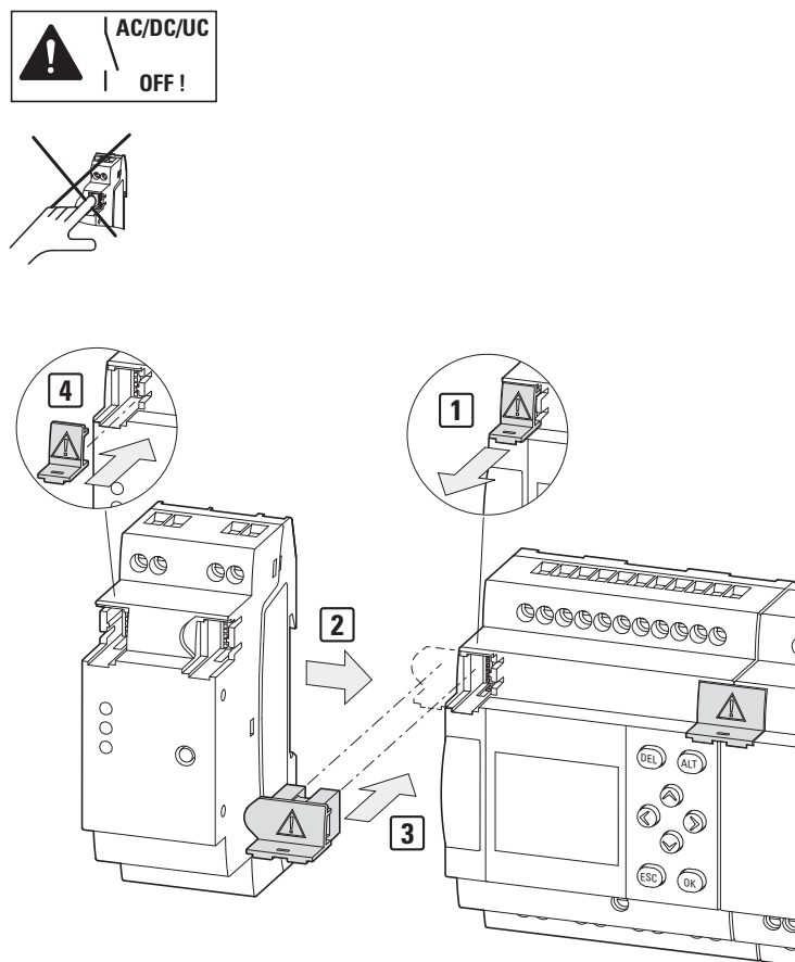
Fig. 11: Montaje del aparato base con módulo de comunicación easy EASY-COM-SWD-C1 como ejemplo
