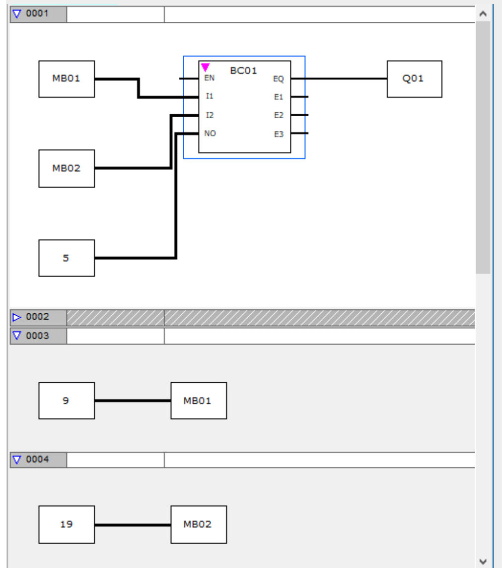
Fig. 207: Proyecto *.e80 con esquema de contactos BC en FBD
