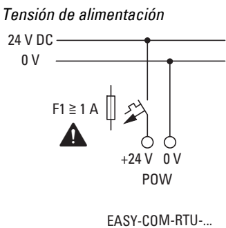
Fig. 351: Conectar la tensión de alimentación EASY-COM-RTU-...
