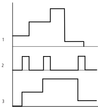
Fig. 214: Diagrama de comportamiento módulo de datos
