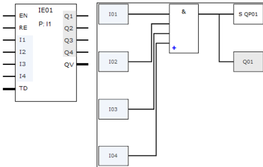
Fig. 266: Transferencia de los estados de entradas y salidas entre el programa principal y el programa de interrupción
