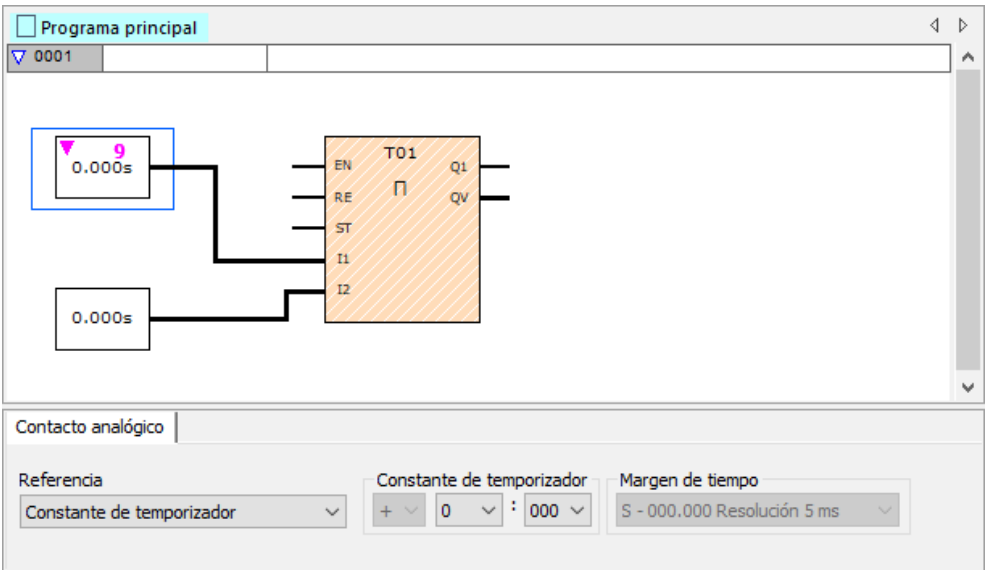
Fig. 122: Vista Programación: constante de temporizador seleccionada en la entrada del módulo I1 y entrada de teclado no confirmada del valor <9>
