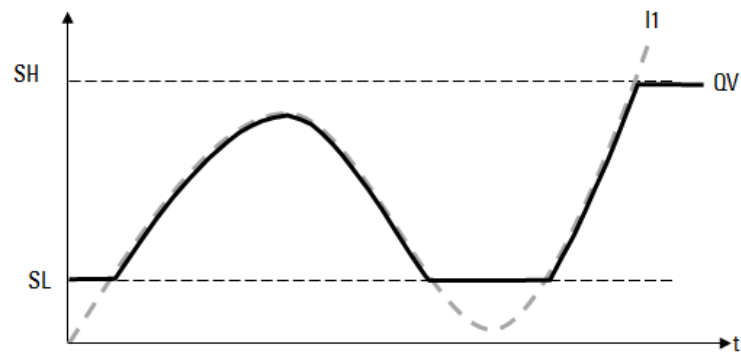
Fig. 206: Figura: Recorte de los valores de entrada según los límites establecidos
