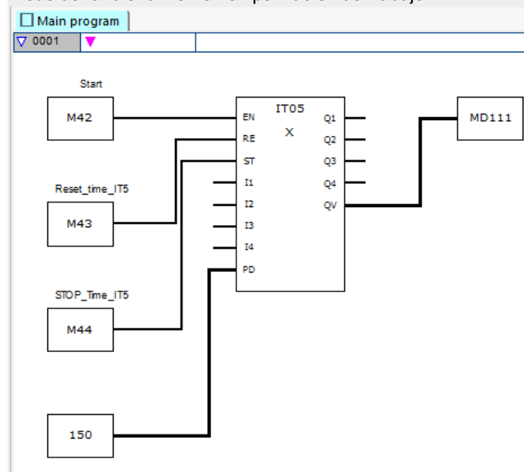
Fig. 270: easySoft 8 Programa principal controlado por tiempo
