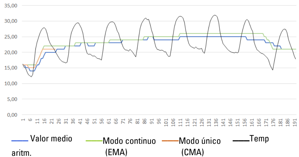
Fig. 182: Curva característica de ejemplo de la medición de temperatura por horas, durante 7 días
