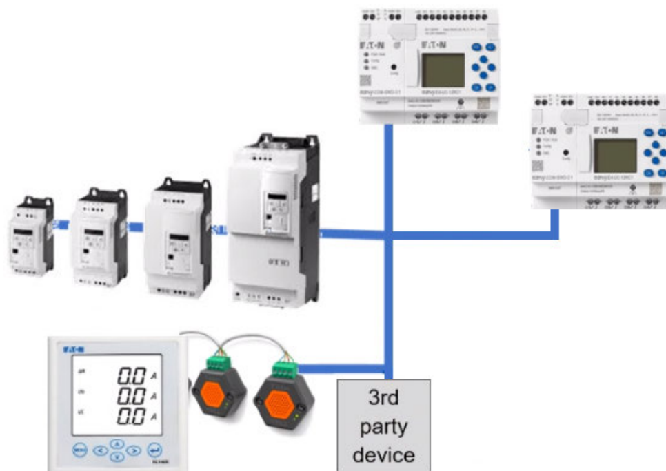
Fig. 348: Sinóptico: easyE4 como maestro Modbus RTU se comunica con DE1, DC1, DG1, DA1, easyE4 como esclavo Modbus RTU y otros aparatos
