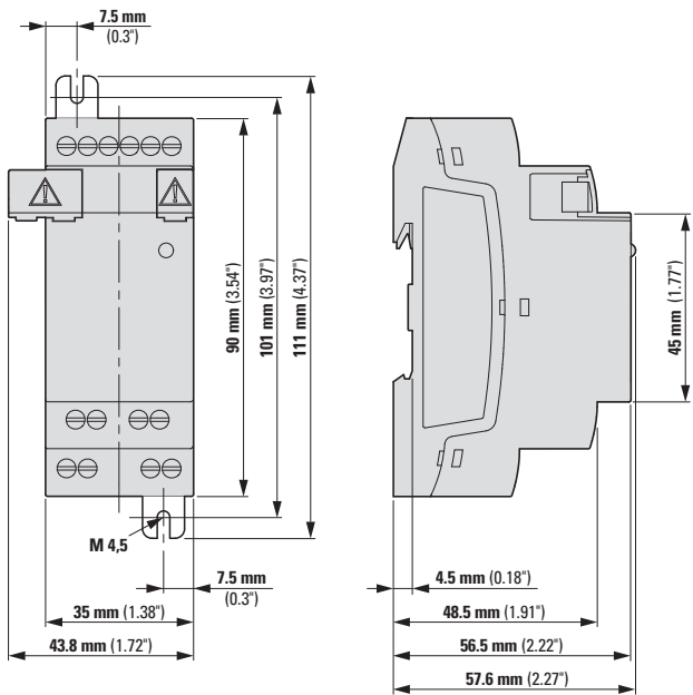
Fig. 400: Dimensiones en mm (pulgadas) ampliaciones 2 ud. división
