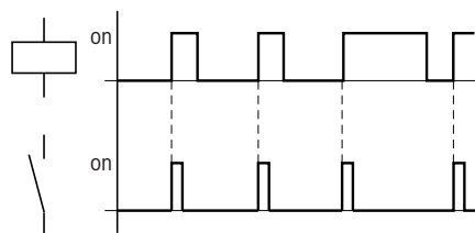
Fig. 102: Diagrama de comportamiento "impulso de ciclo" con flanco positivo
