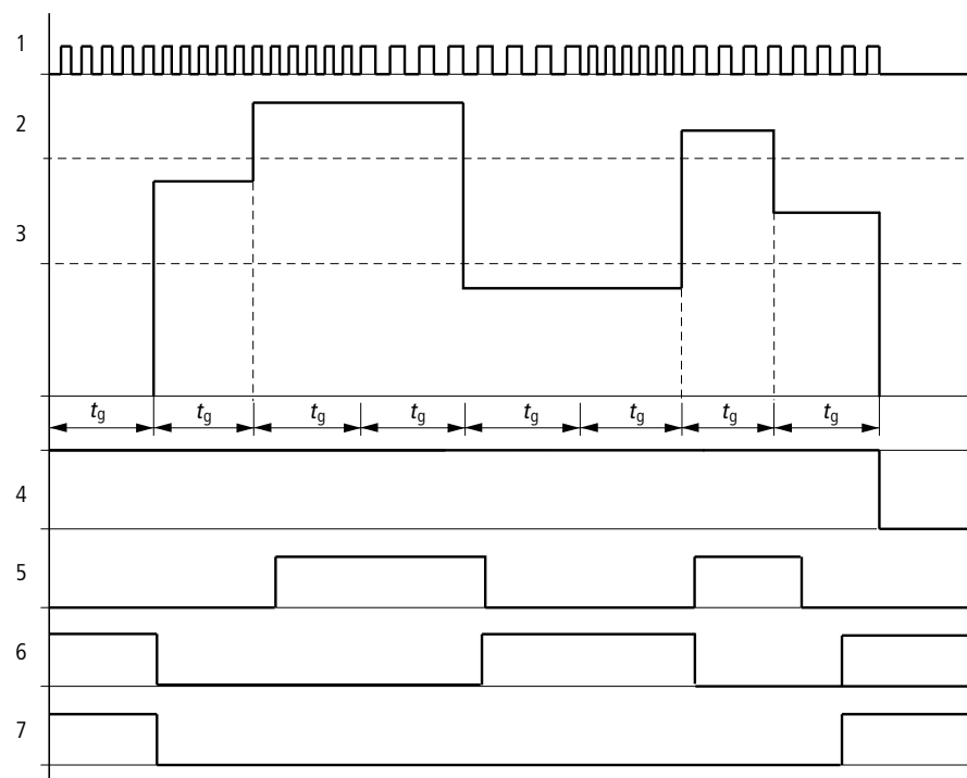
Fig. 173: Diagrama de comportamiento contador de frecuencia
