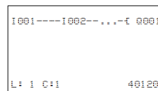
Fig. 84: Esquema de contactos con entradas I01, I02 y salida Q1
