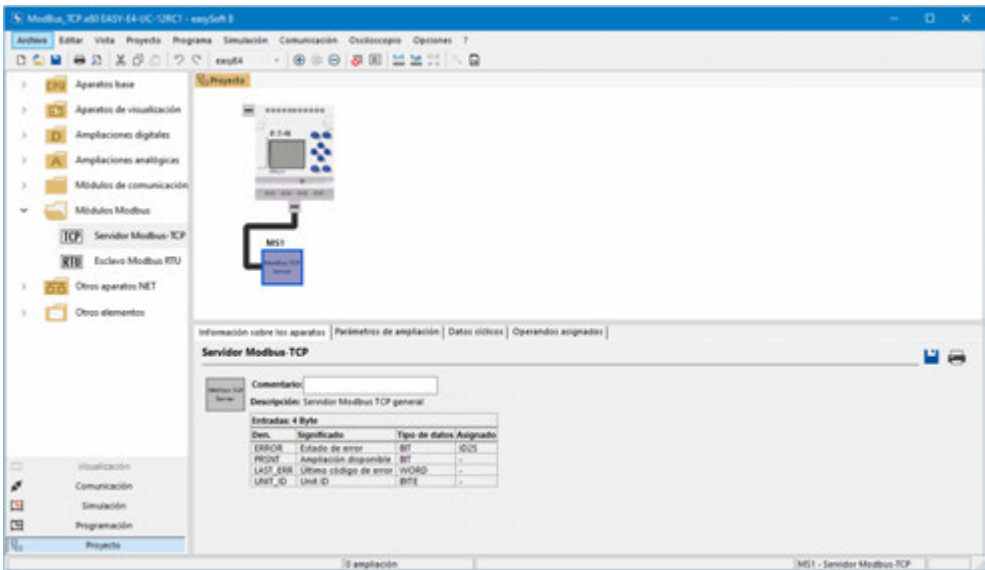
Fig. 384: Interface de trabajo con aparato base y módulos de servidor Modbus-TCP
