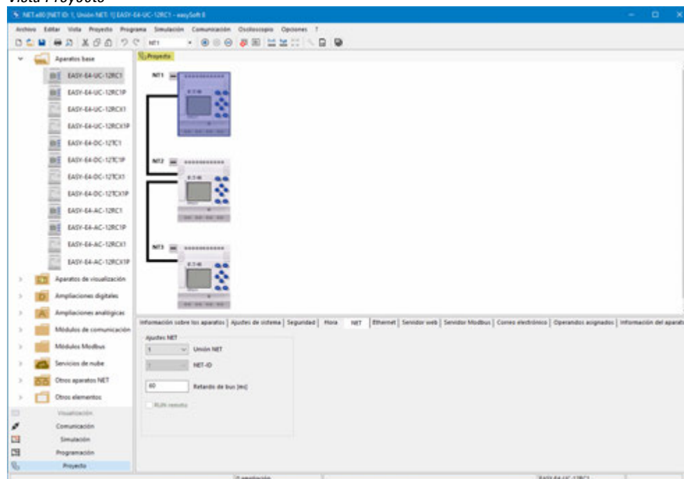
Fig. 315: Configuración NET con el proyecto y el programa
