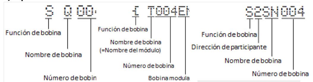
Fig. 107: Bobina de relé "Salida Q"
