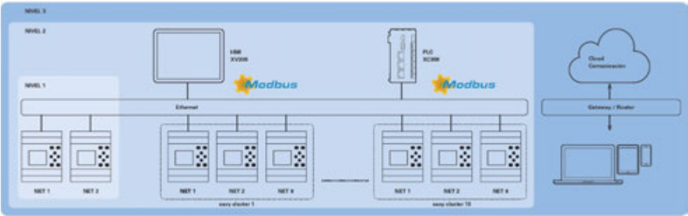
Fig. 318: Sinóptico NET
