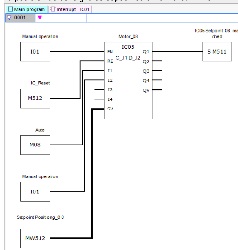
Fig. 262: easySoft 8 Programa principal Transmisor de valores incremental
