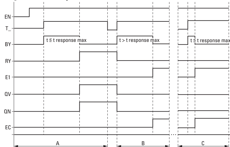
Fig. 242: Diagrama de comportamiento contador de frecuencia
