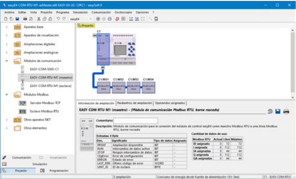
Fig. 352: Área de trabajo con aparato base y módulo de comunicación maestro EASY-COM-RTU-M1
