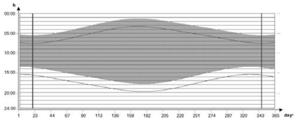
Fig. 169: Offset; O1=-2; O2=-2; Q1=1 se conecta 2 horas antes de la salida del sol y 2 horas antes de la puesta del sol
