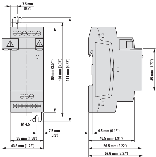
Fig. 401: Dimensiones en mm (Inch)
