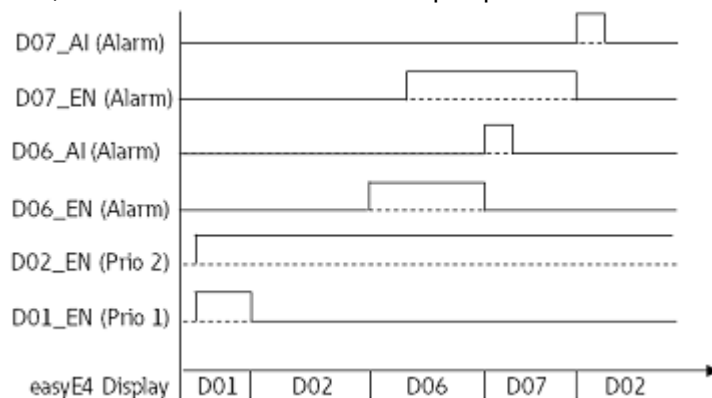
Fig. 226: Diagrama de comportamiento Visualización de texto
