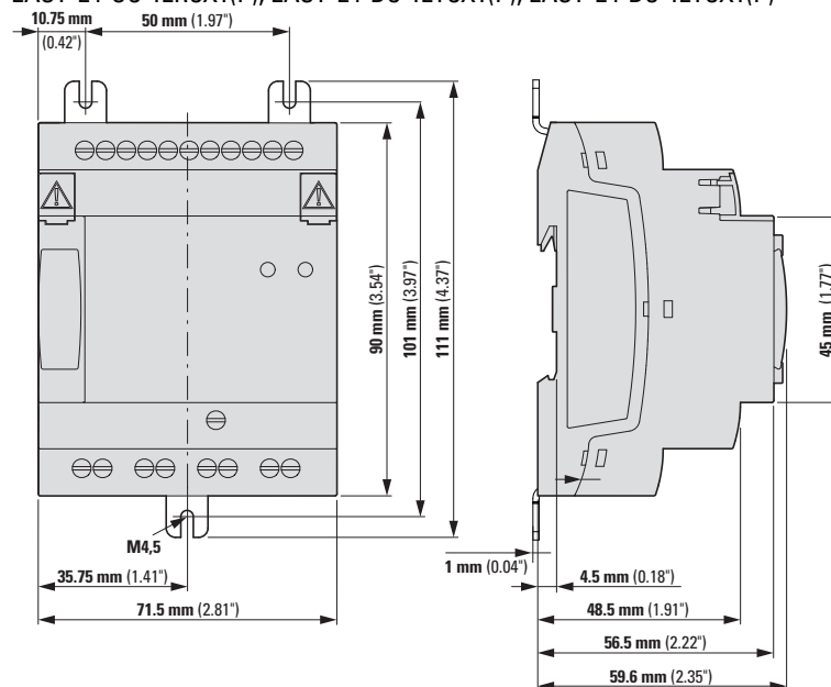
Fig. 398: Dimensiones en mm (pulgadas) de los aparatos base EASY-E4-...-12...CX1(P)
