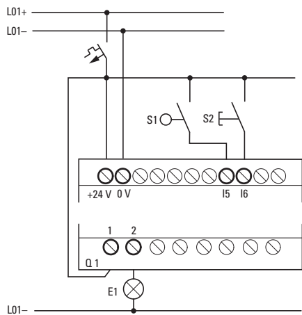
Fig. 291: Cableado p. ej. con EASY-E4-UC-...
