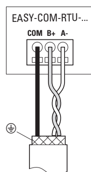
Fig. 350: EASY-COM-RTU-...Conexión de las salidas
