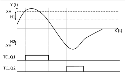
Fig. 205: Diagrama de comportamiento Regulador de tres vías
