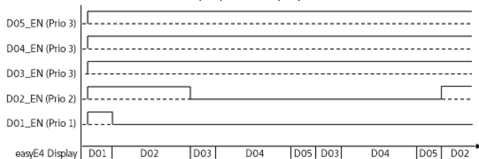
Fig. 227: Diagrama de comportamiento Visualización de texto con los módulos de texto que tienen la misma prioridad 3
