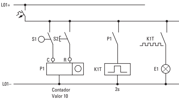
Fig. 290: Cableado fijo con relé
