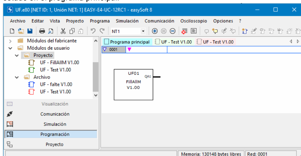
Fig. 284: easySoft 8 con catálogo a la izquierda, directorio Módulos de usuario/Proyecto y Módulos de usuario/Archivo con distintos contenidos UF-BETest V1.00
