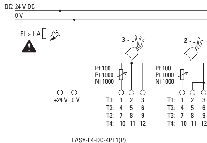
Fig. 30: Conexión de las entradas analógicas EASY-E4-DC-4PE1(P)
