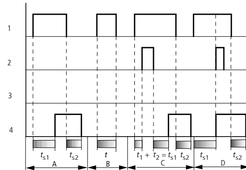
Fig. 149: Diagrama de comportamiento relé temporizador, temporización de trabajo y reposo
