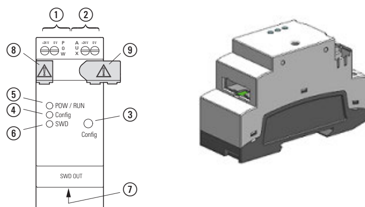
Fig. 344: Versión del aparato con 2TE
