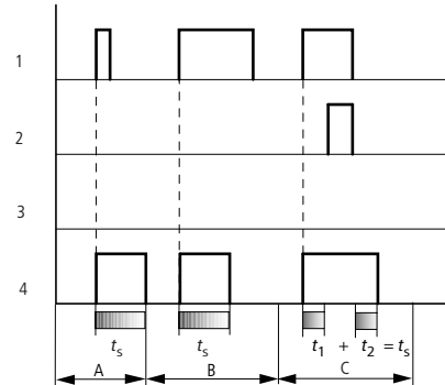
Fig. 150: Diagrama de comportamiento, generación de un impulso a partir de una señal 1
