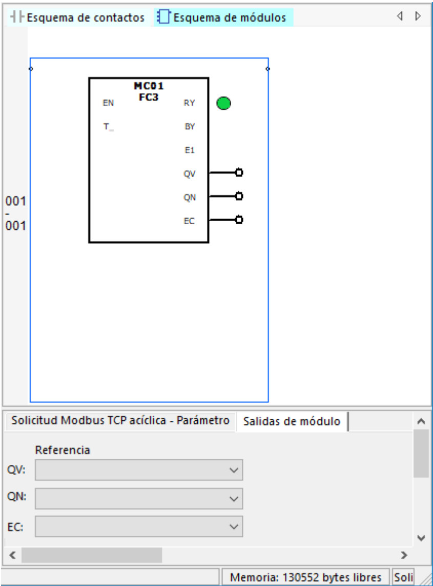
Fig. 241: Registro Salidas de módulo
