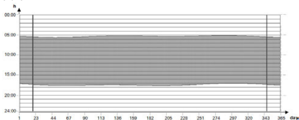
Fig. 165: Offset; O1=-2; O2=2; Q1=1 se conecta 2 horas antes de la salida del sol y 2 horas tras la puesta del sol
