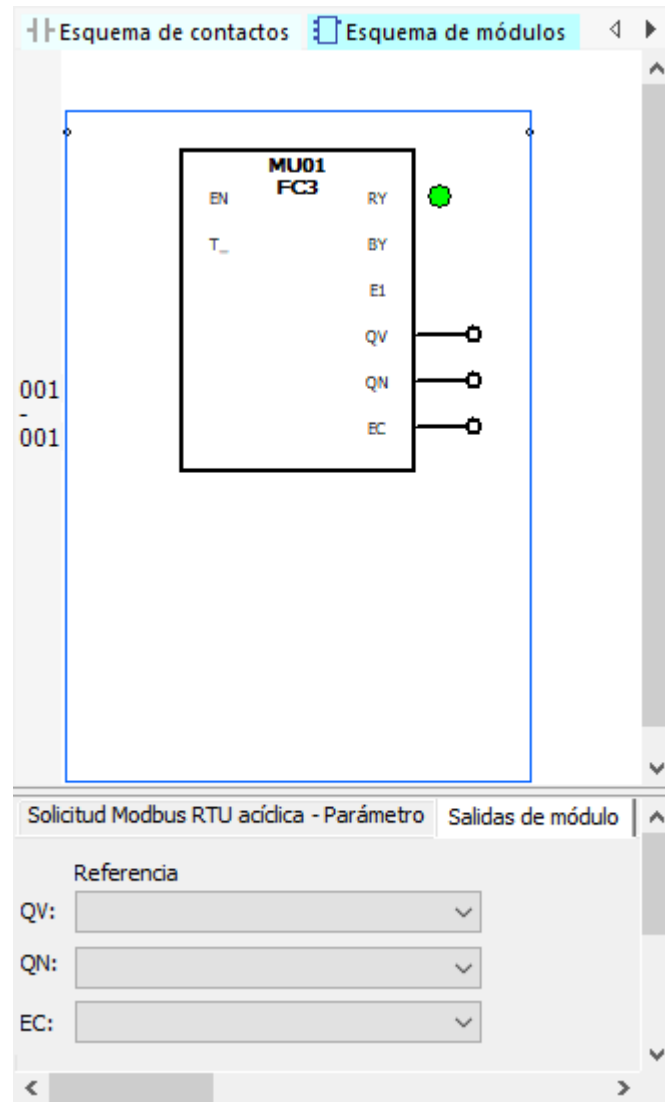
Fig. 251: Registro Salidas de módulo
