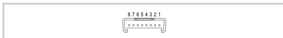
Abb. 16 SWD-Schnittstelle (Stiftleiste, 8-polig)
