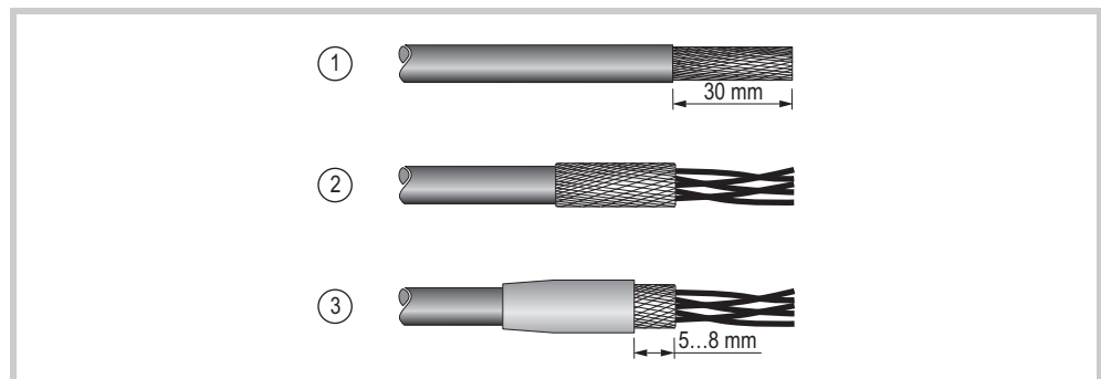
Abb. 5 Kabelschirm anschliessen
