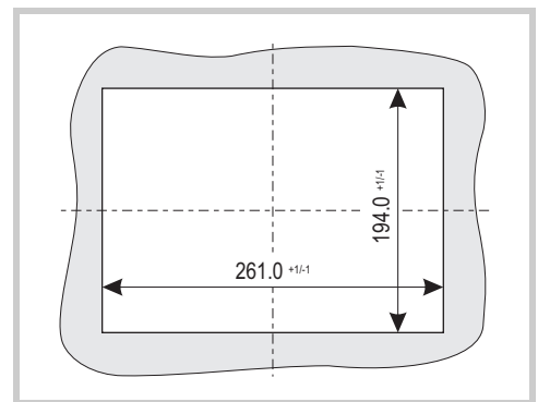
Abb. 24 Einbauausschnitt für 8,4"-Geräte
