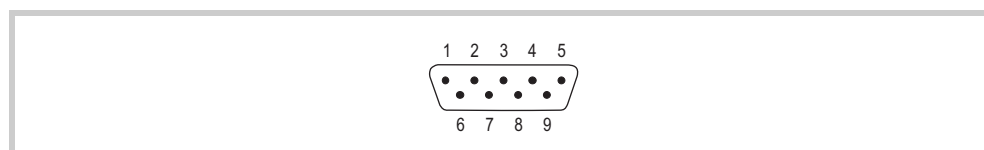
Abb. 21 RS485-Schnittstelle (9-polig, D-Sub, male, UNC)
