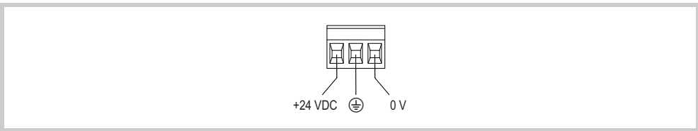
Abb. 8 Steckverbinder Phoenix Contact MSTB 2.5/3-ST-5.08 (Ansicht von der Verdrahtungsseite)
