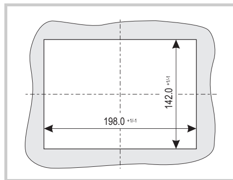
Abb. 23 Einbauausschnitt für 5,7"-Geräte
