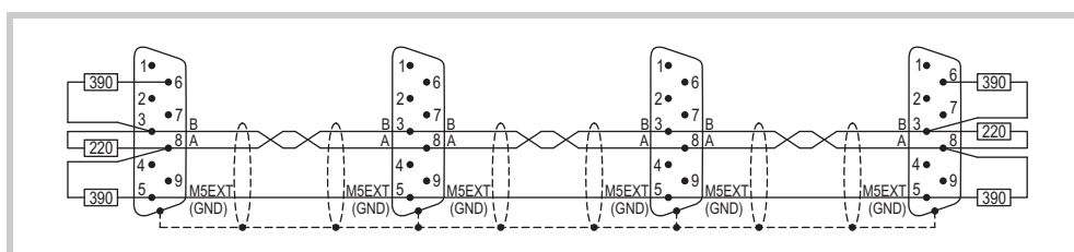
Abb. 20 Bussegment mit vier Busteilnehmern
