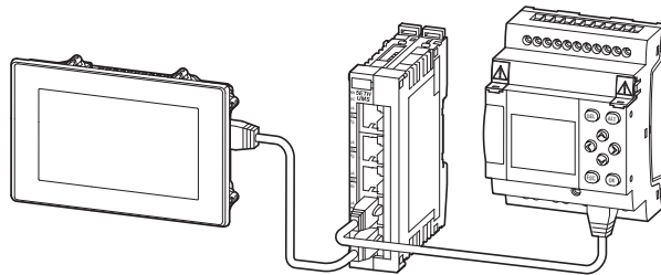
Abb. 55: Ethernet-Verbindung der Geräte RTD und easyE4 über einen Ethernet-Switch
