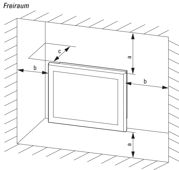
Abb. 5: Einbauabstand
