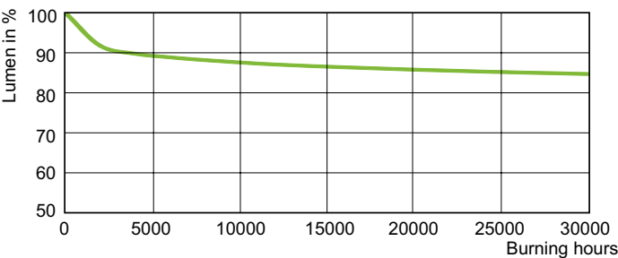
Lumen Maintenance Diagram - MASTER SON PIA Plus 50W E27
