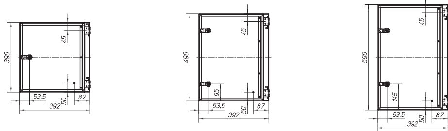
Tueren_Kombi_BS_GR_425
