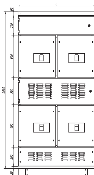
4xNZM4
