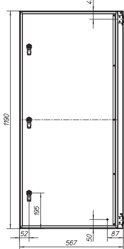
Tueren_Kombi_BS_GR_600
