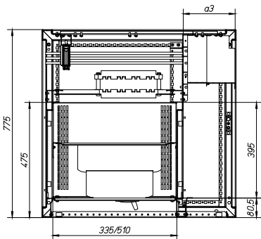
XF_NZM1_3_F4_800_D
