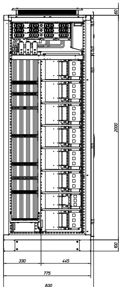
XF_4b_W800_Katalog
