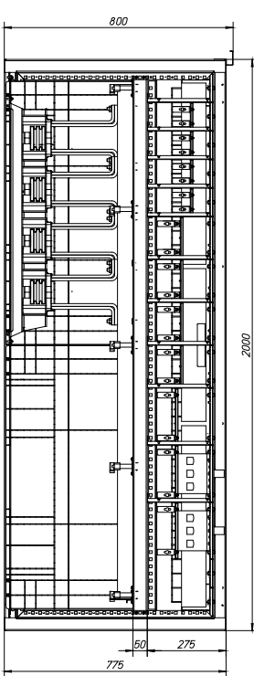
XF_NZM1_3_F4_800_S_oMS
