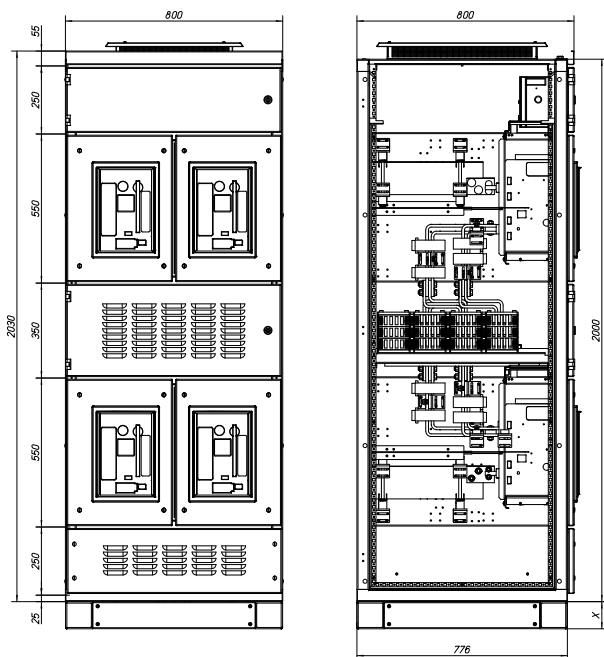
XP_4xIZMX16_stackedACB_Mas
