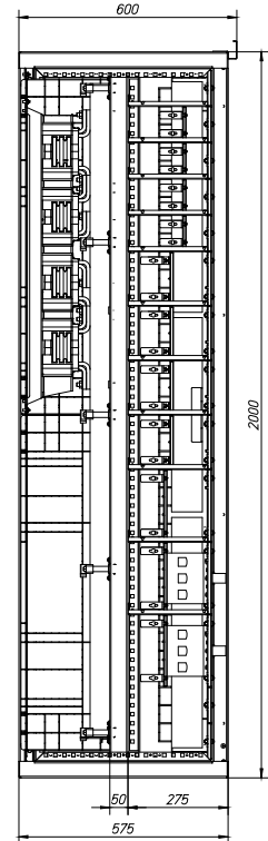
XF_NZM1_3_F4_600_S_oMS
