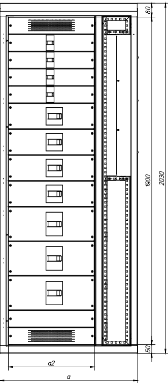
XF_NZM1_3_F4_800_V_mFP
