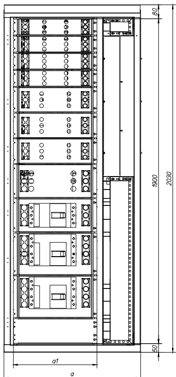
XF_NZM1_3_F2b_600_V
