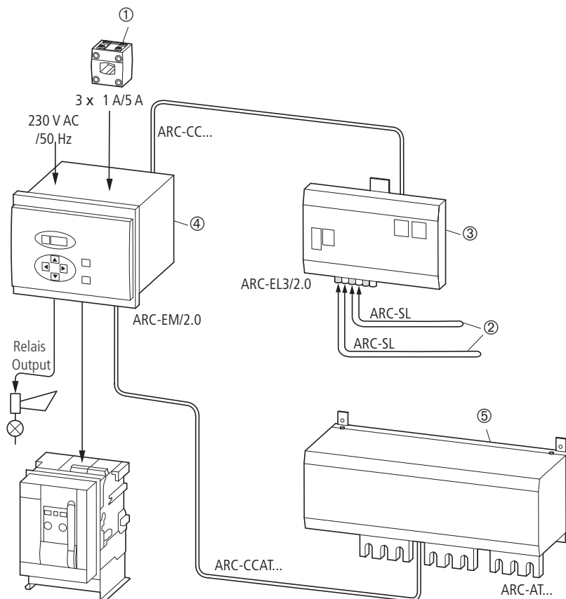
ARCON_Komponenten
