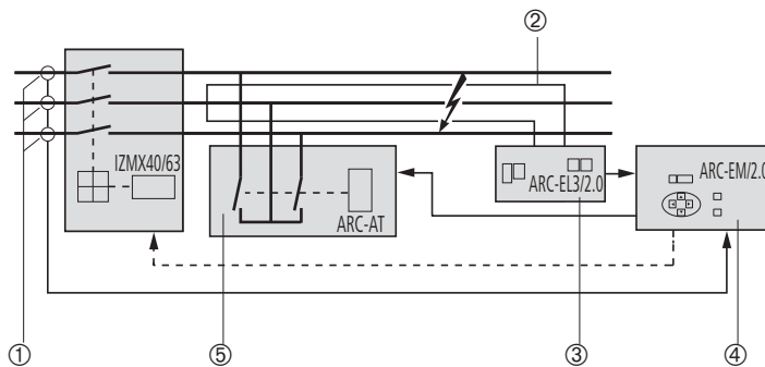
ARCON_Funktionsprinzip
