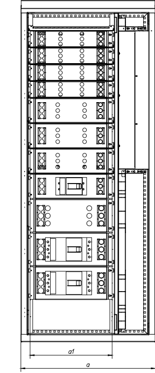
XF_NZM1_3_F4_600_V_mFP
