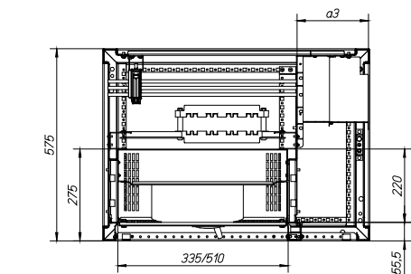
XF_NZM1_3_F4_600_D
