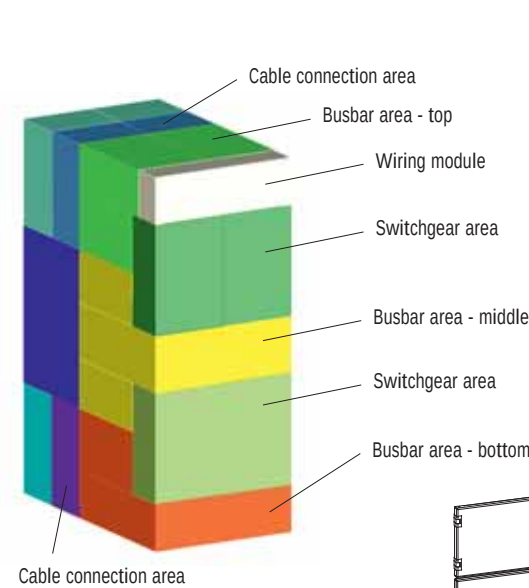
XP_Funktionsraeume_4x_stacked
