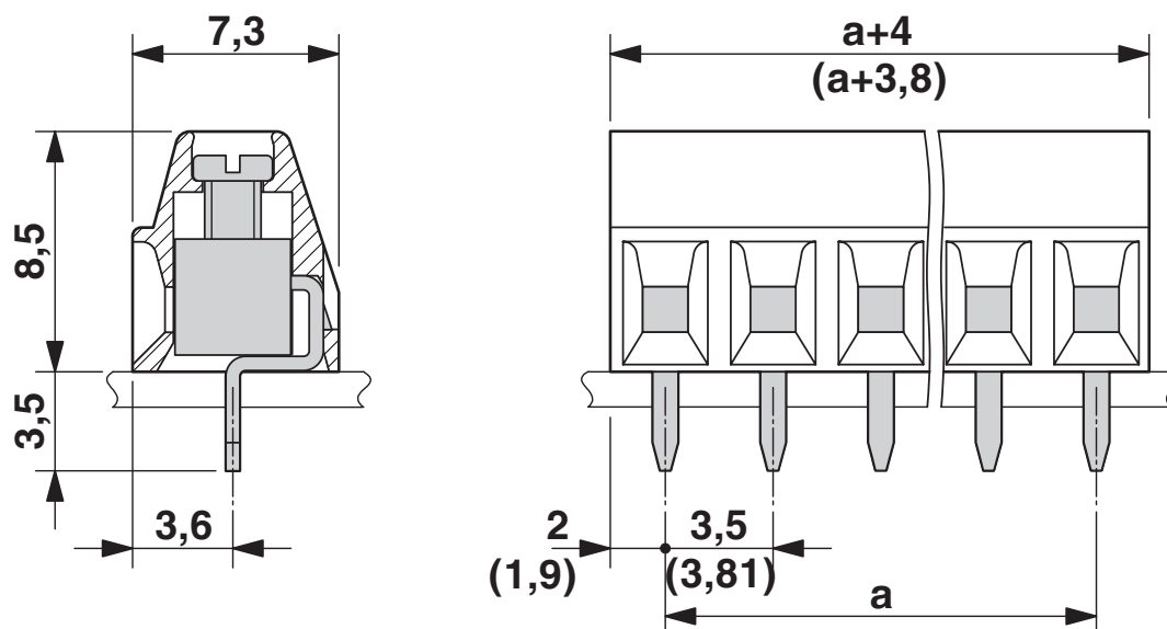
Maatschets
