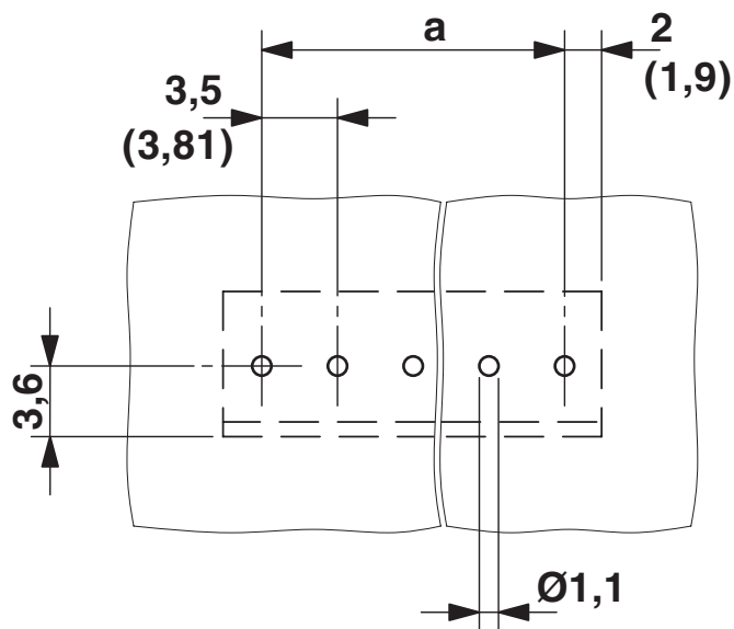
boorsjabloon/soldeerpadgeometrie
