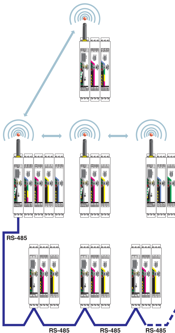
functietekening
