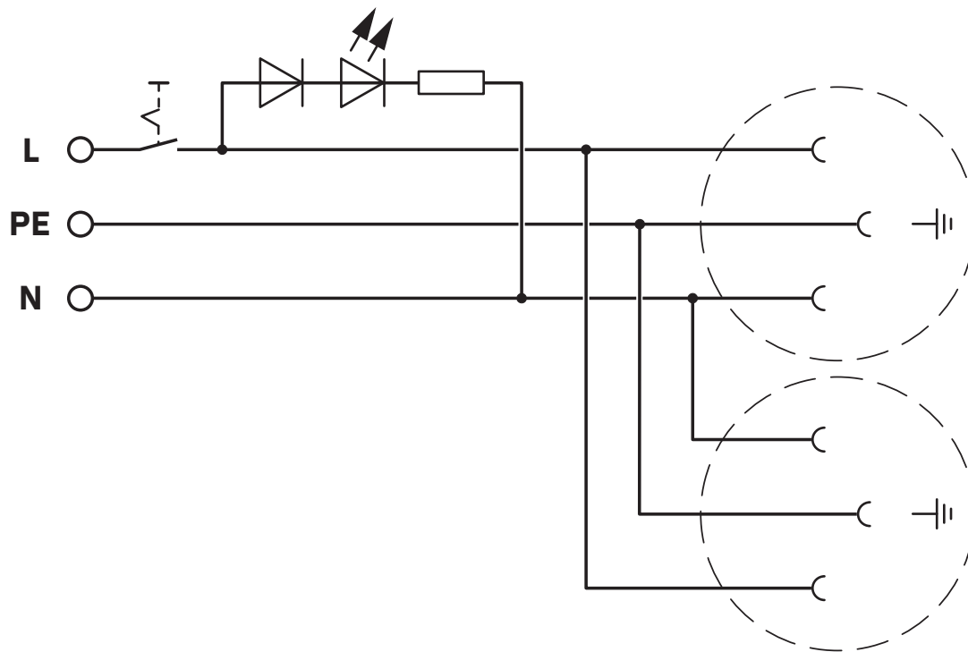
schakelschema
