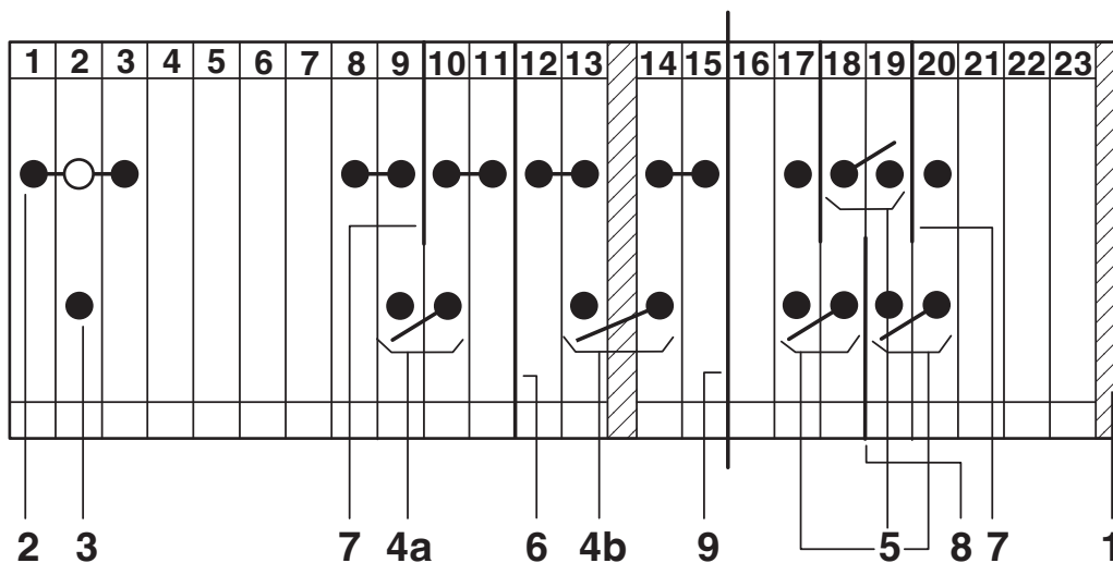
schakelschema
