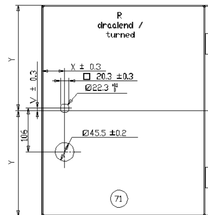
HANDGRIEP / HANDLE
