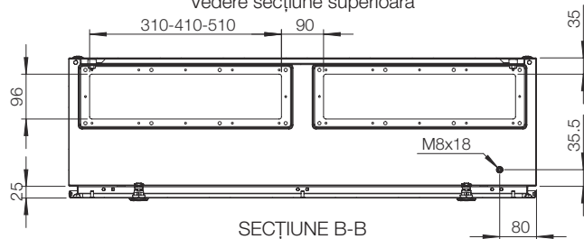
SECȚIUNE B-B
