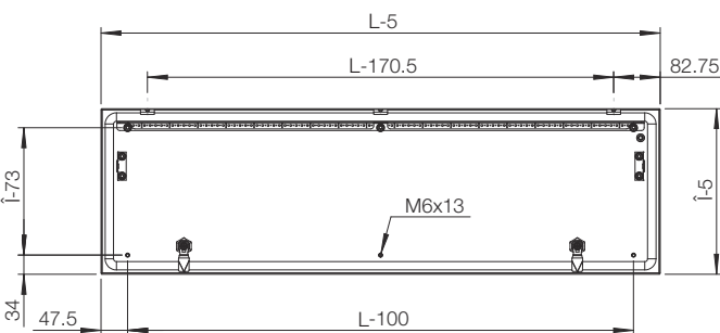
Vedere interioară ușă panou
