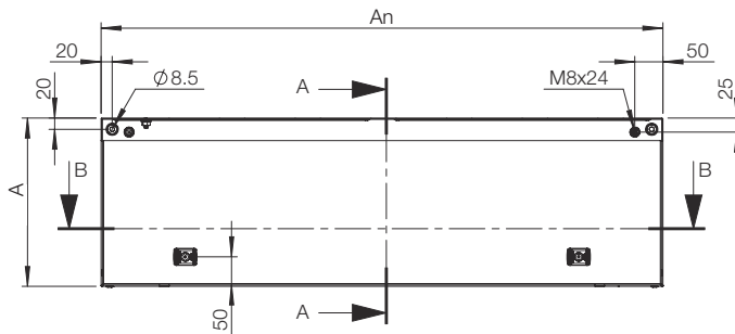
Vista seccional superior
