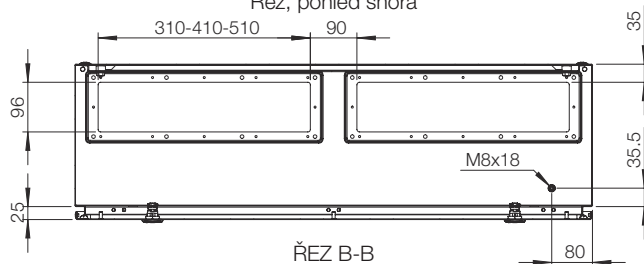
ŘEZ B-B
