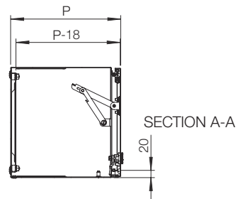
Coupe transversale (latérale)
