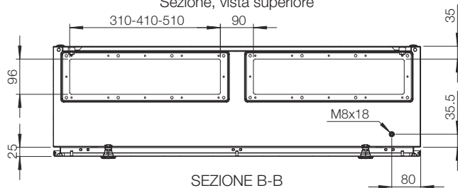
SEZIONE B-B
