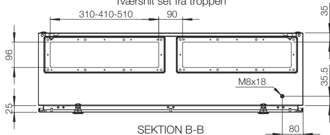
Tværsnit set fra toppen
