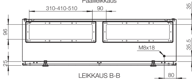
LEIKKAUS B-B
