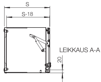
Sivuleikkaus
