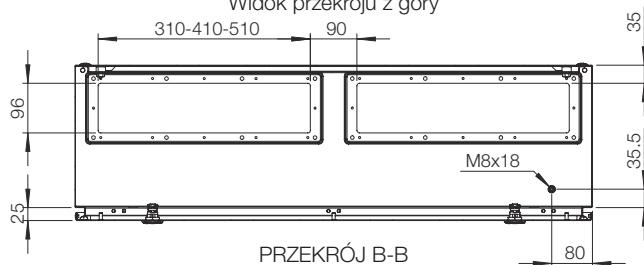
PRZEKRÓJ B-B
