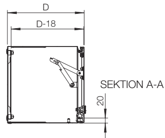
Tværsnit set fra siden
