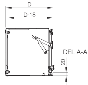
Seksjon side bilde
