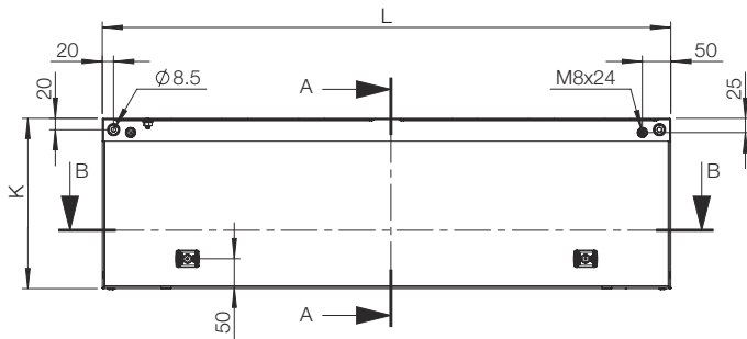
Päälleikkaus
