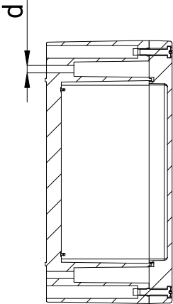
SECTION A-A
