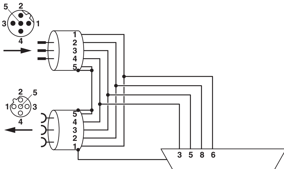
Functieschakelschema SUBCON-PLUS-PROFIB/...M12
