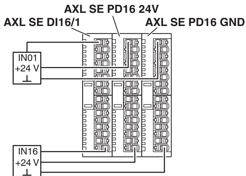
aansluitschema
