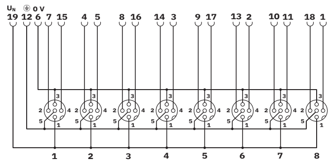
schakelschema
