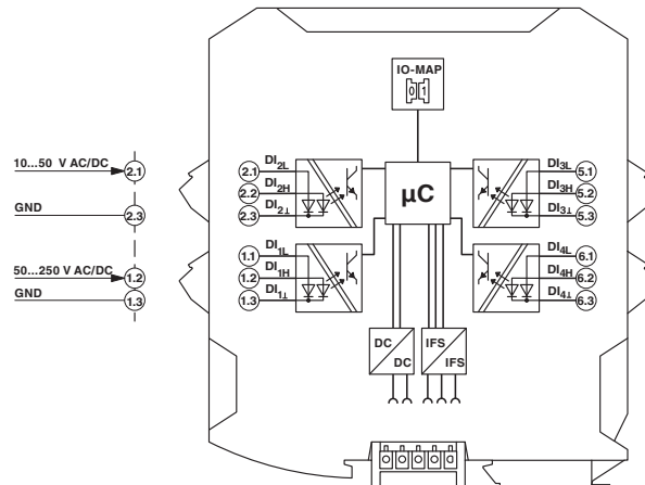
schakelschema
