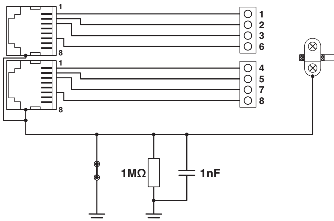
schakelschema
