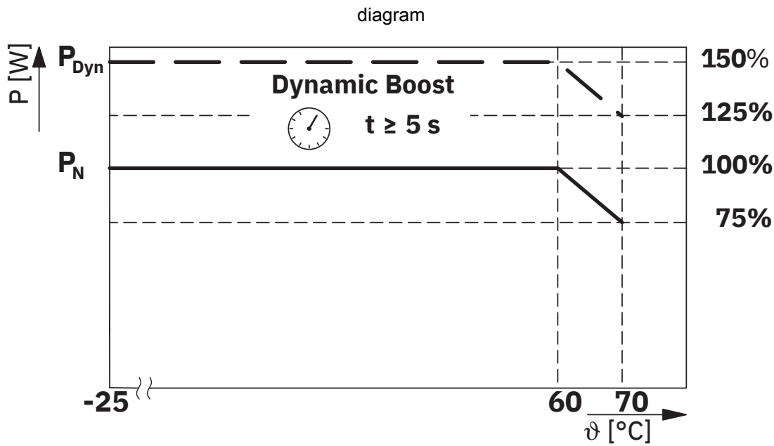
Temperatuurafhankelijke derating
