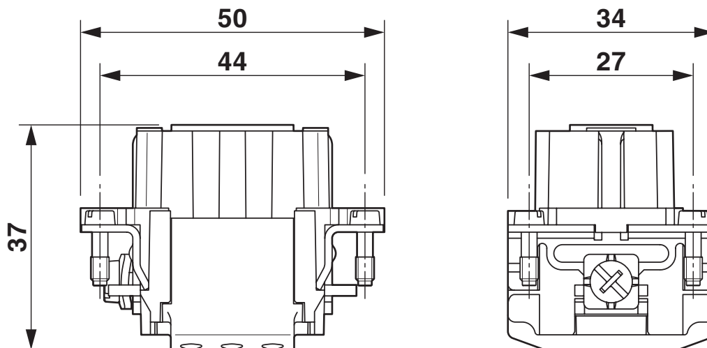
Maatschets
