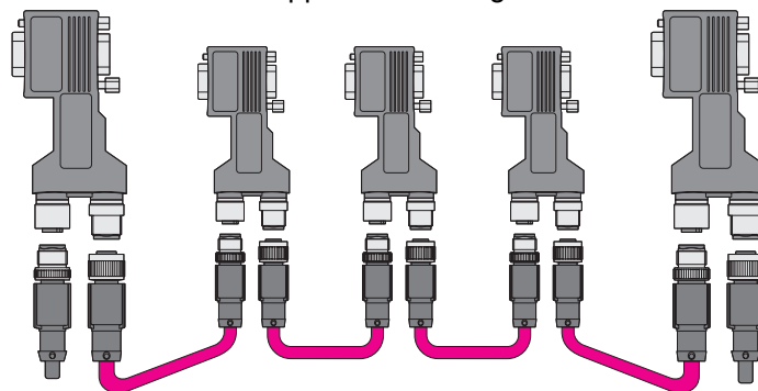
applicatietekening
