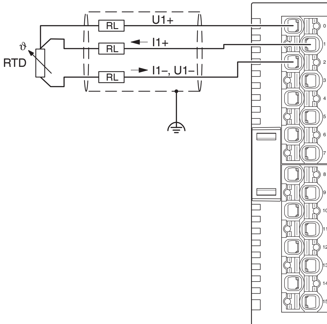
aansluitschema
