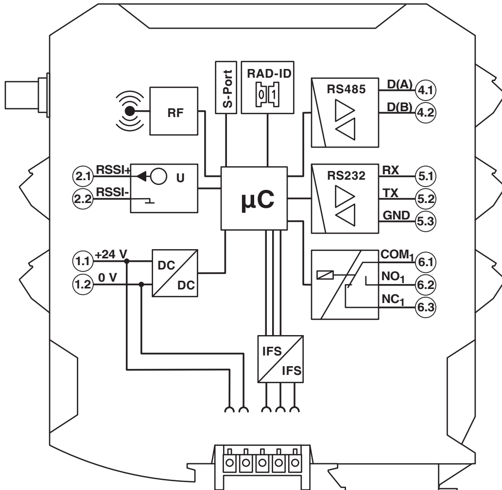
schakelschema
