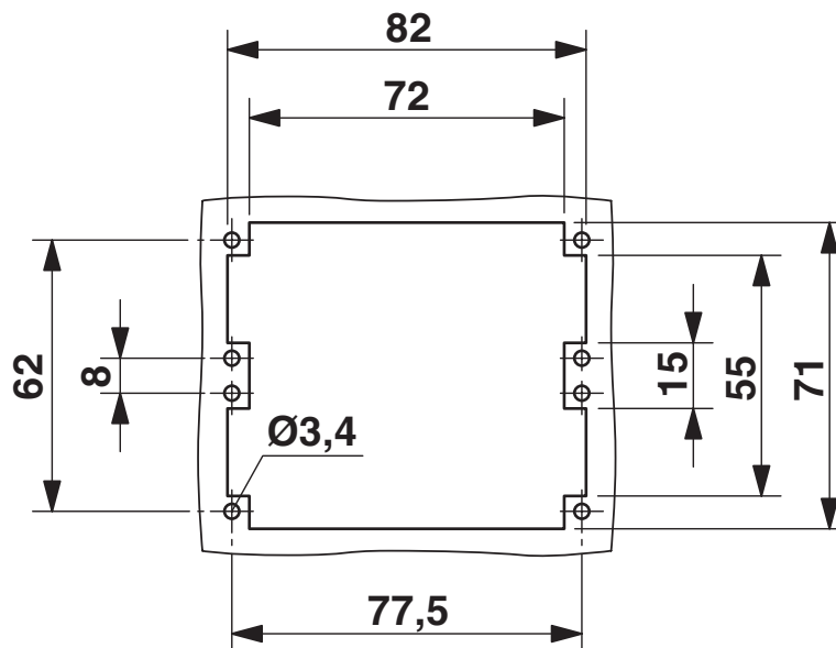
Maatschets
