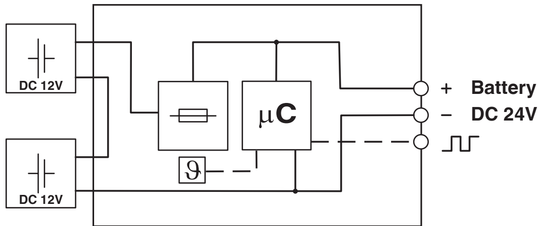
blokschema
