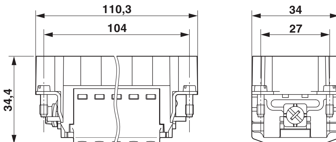
Maatschets
