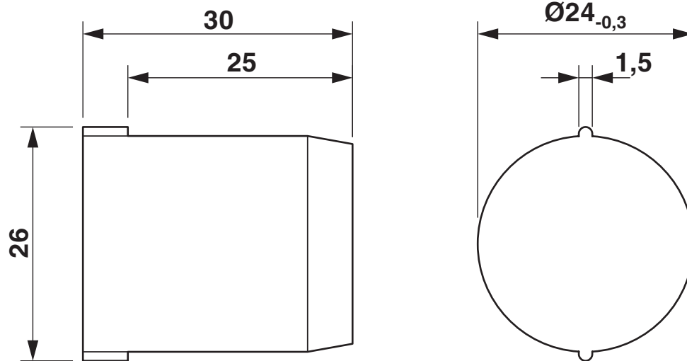
Maatschets
