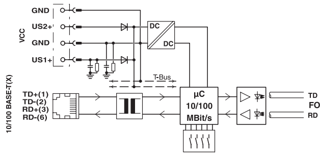
blokschema
