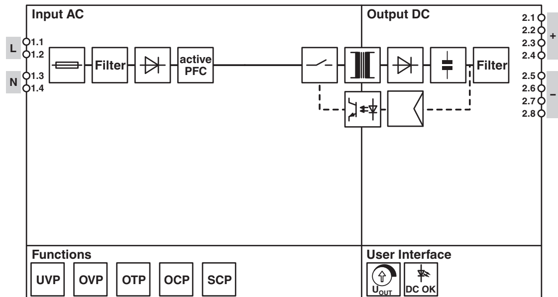
blokschema
