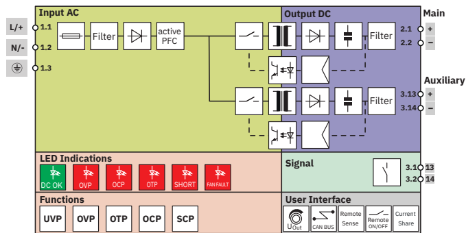
blokschema
