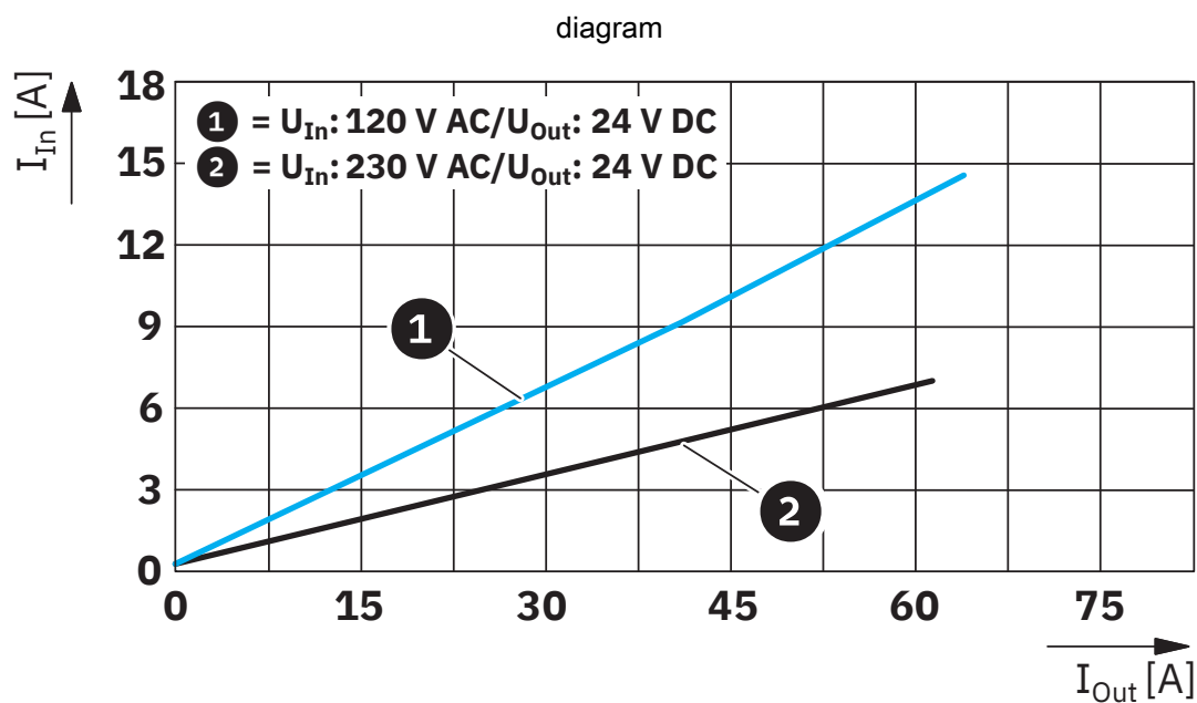
Ingangsstroom/uitgangsstroom
