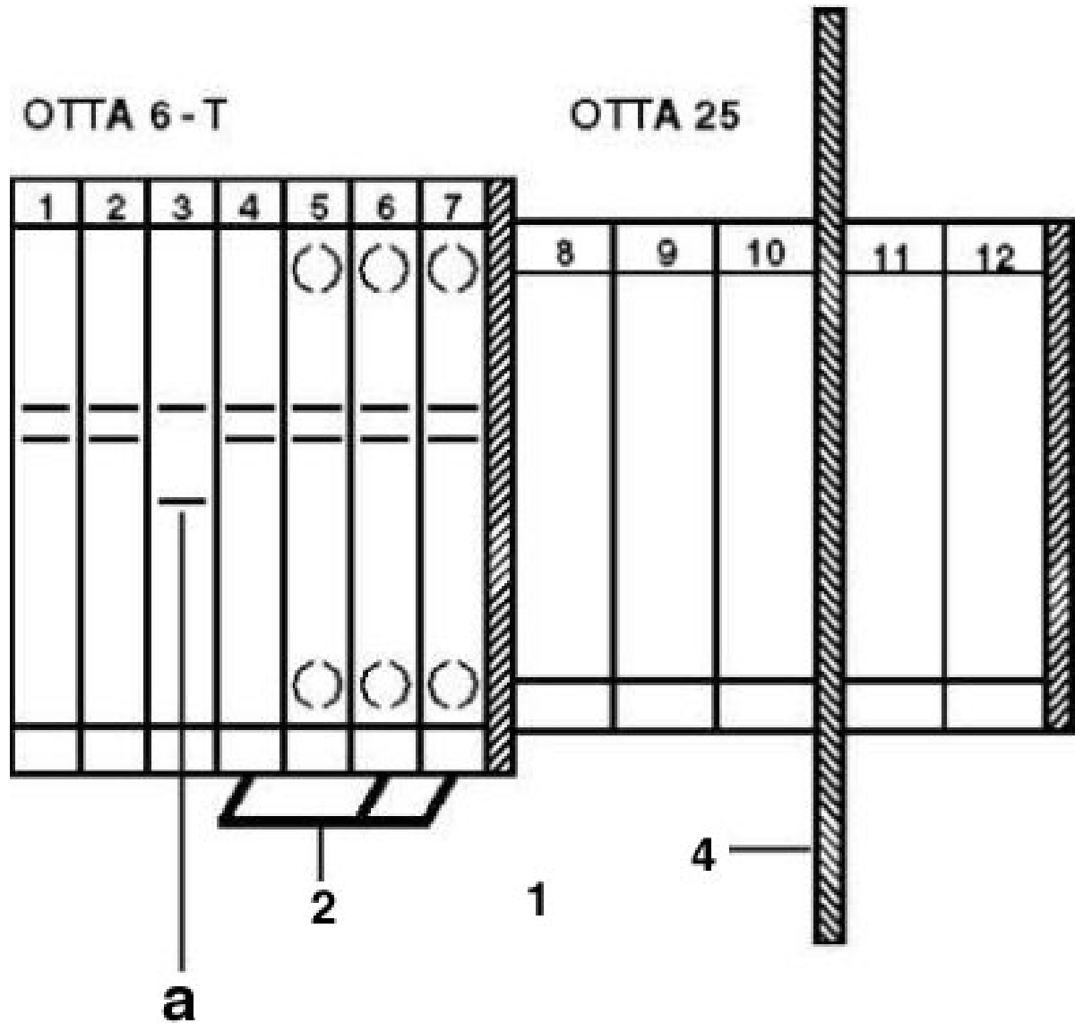
schakelschema
