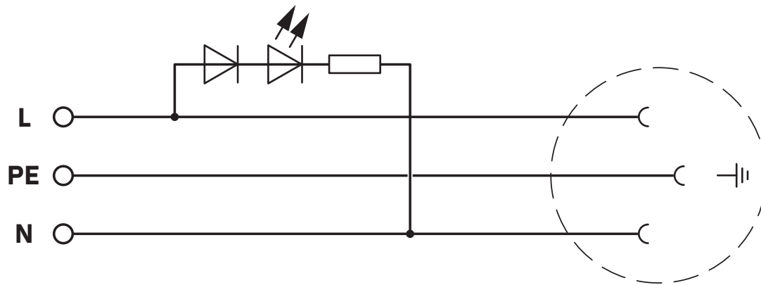
schakelschema
