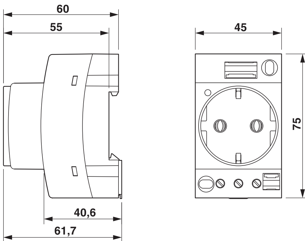
Maatschets
