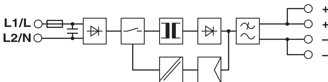
blokschema
