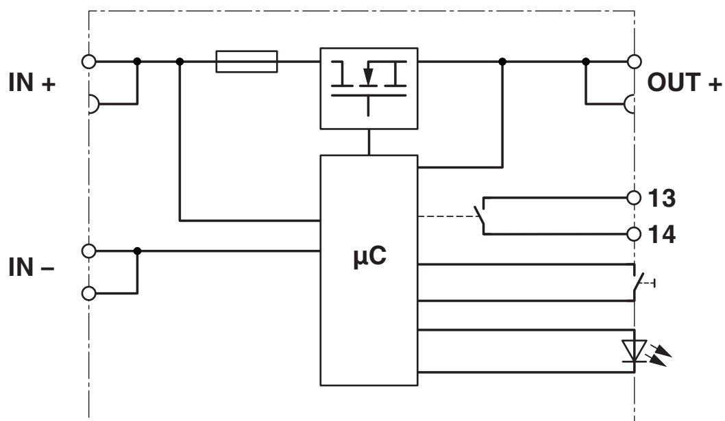
blokschema
