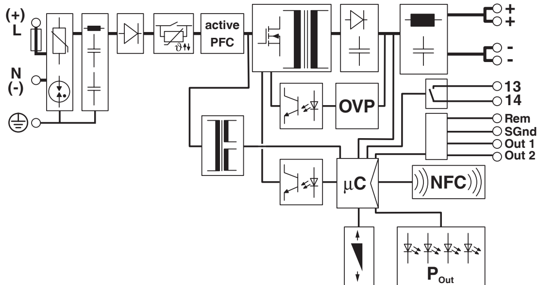
blokschema
