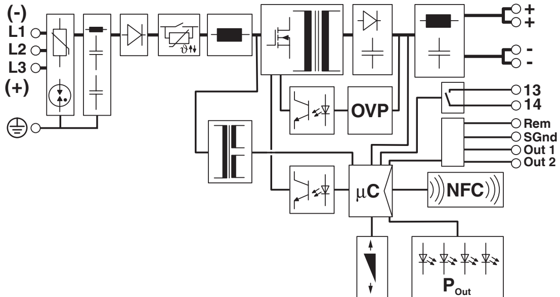
blokschema
