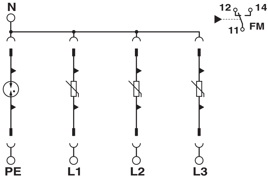
schakelschema
