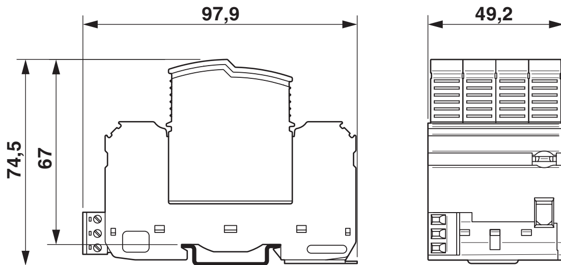
Maatschets
