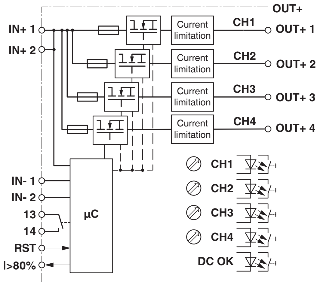
blokschema
