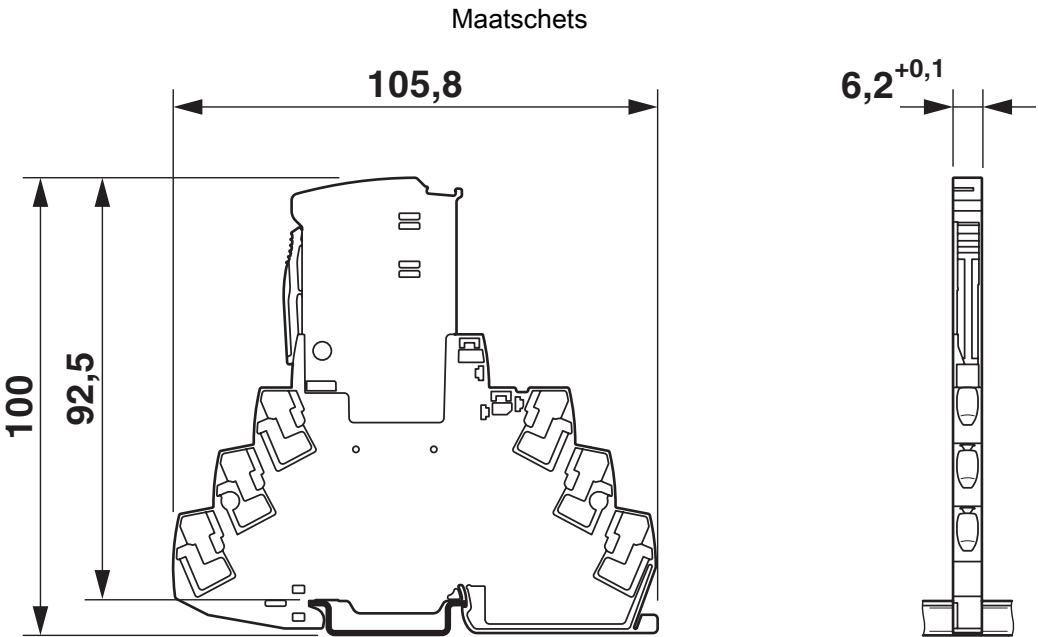
schematekening
