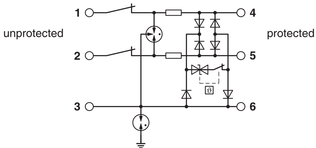
schakelschema
