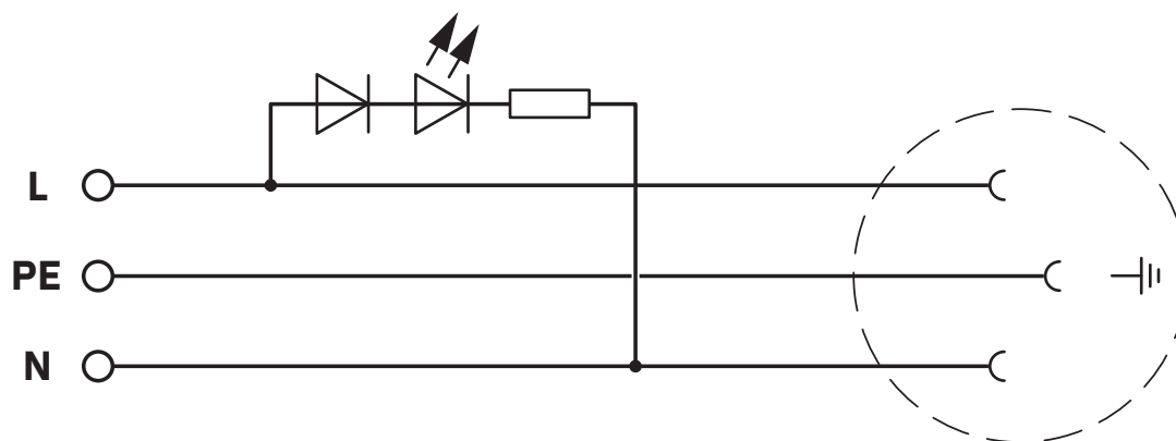
schakelschema
