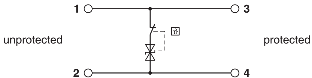
schakelschema
