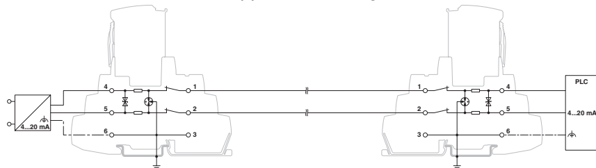
applicatietekening
