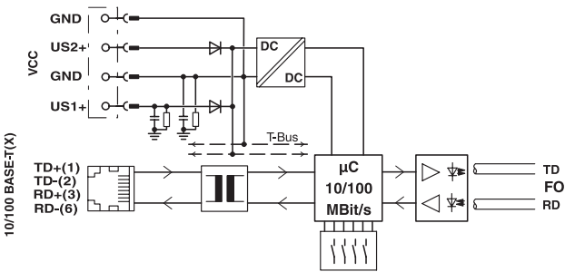
blokschema
