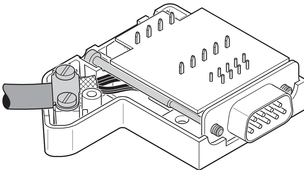
schematekening
