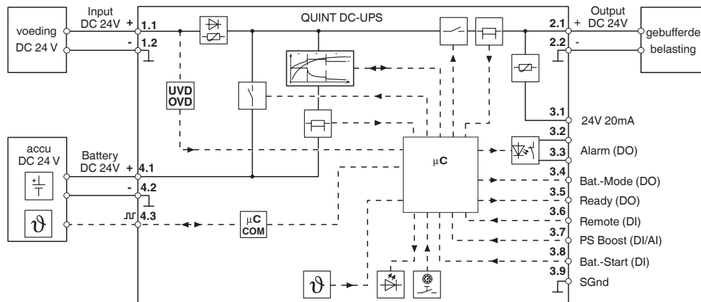
blokschema
