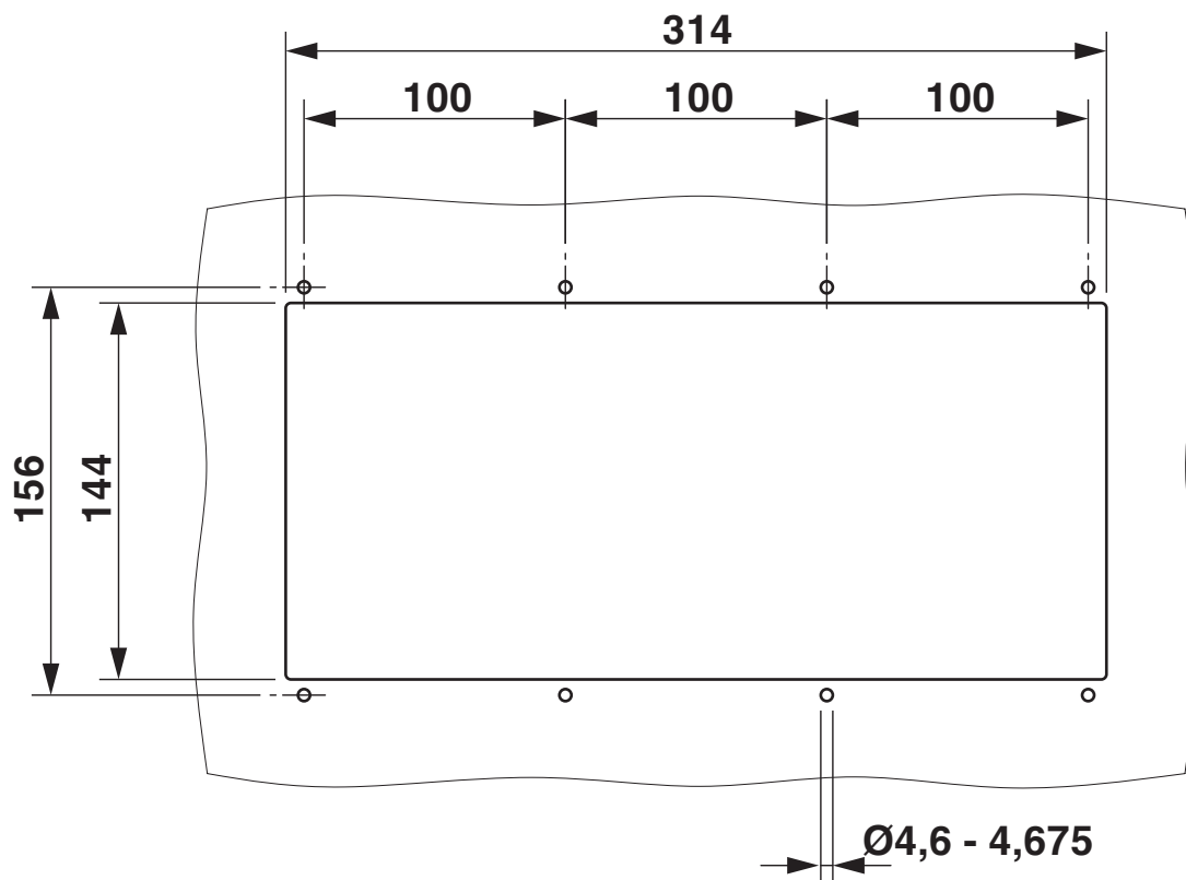
Tekening wanduitsparing
